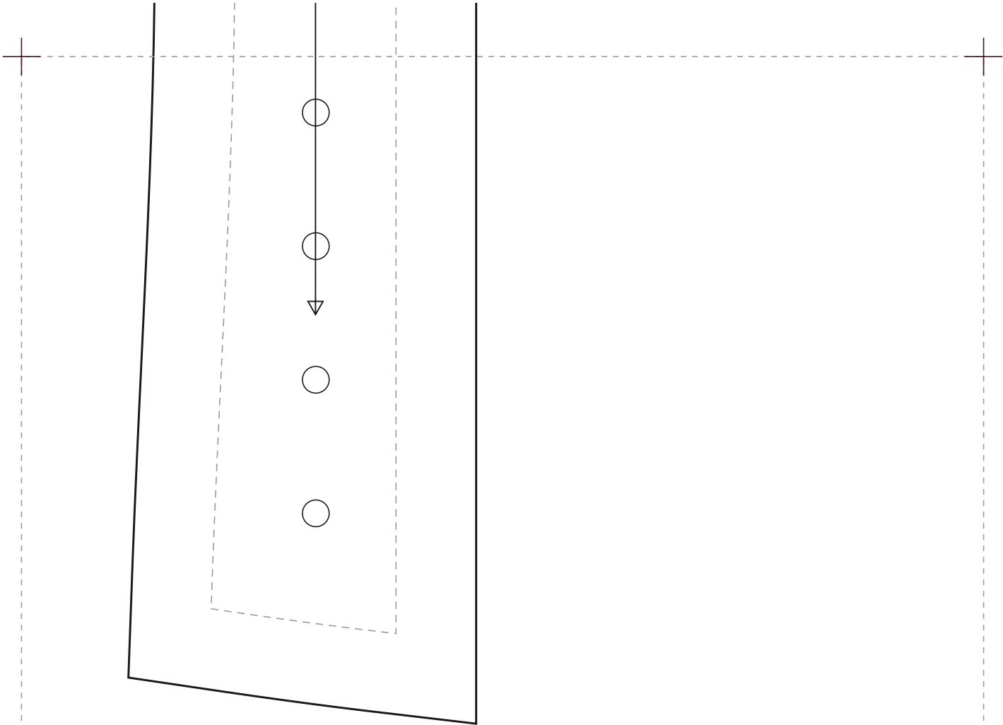
CORSÉ 072 · Sobre Busto Escote Recto · 10 Paneles · Cordón Adelante · escala 1:1 · 95,9 × 88,6 cm
