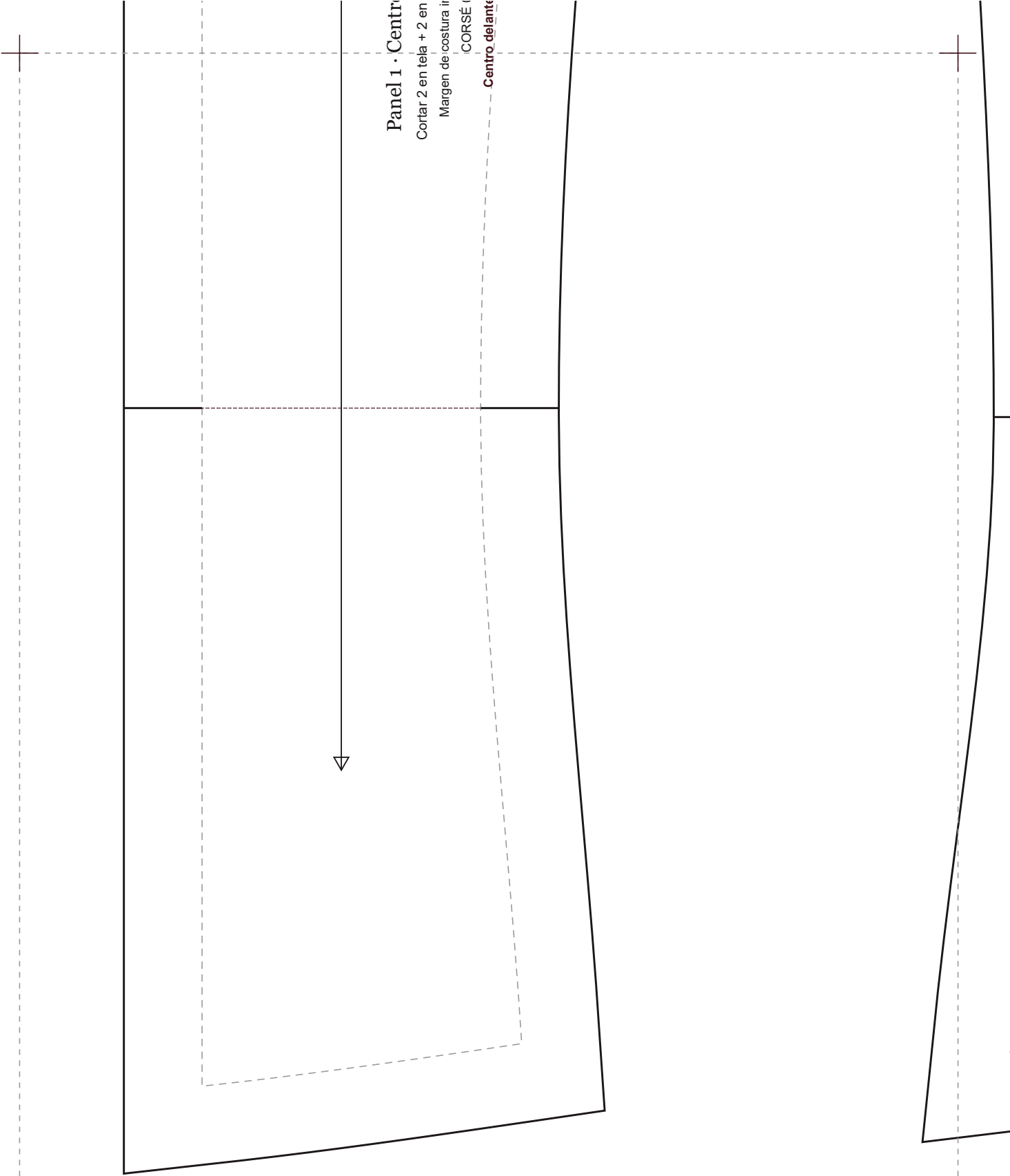
CORSÉ 083 · Sobre Busto Escote en V Suave · 6 Paneles · escala 1:1 · 89,1 × 48,2 cm
