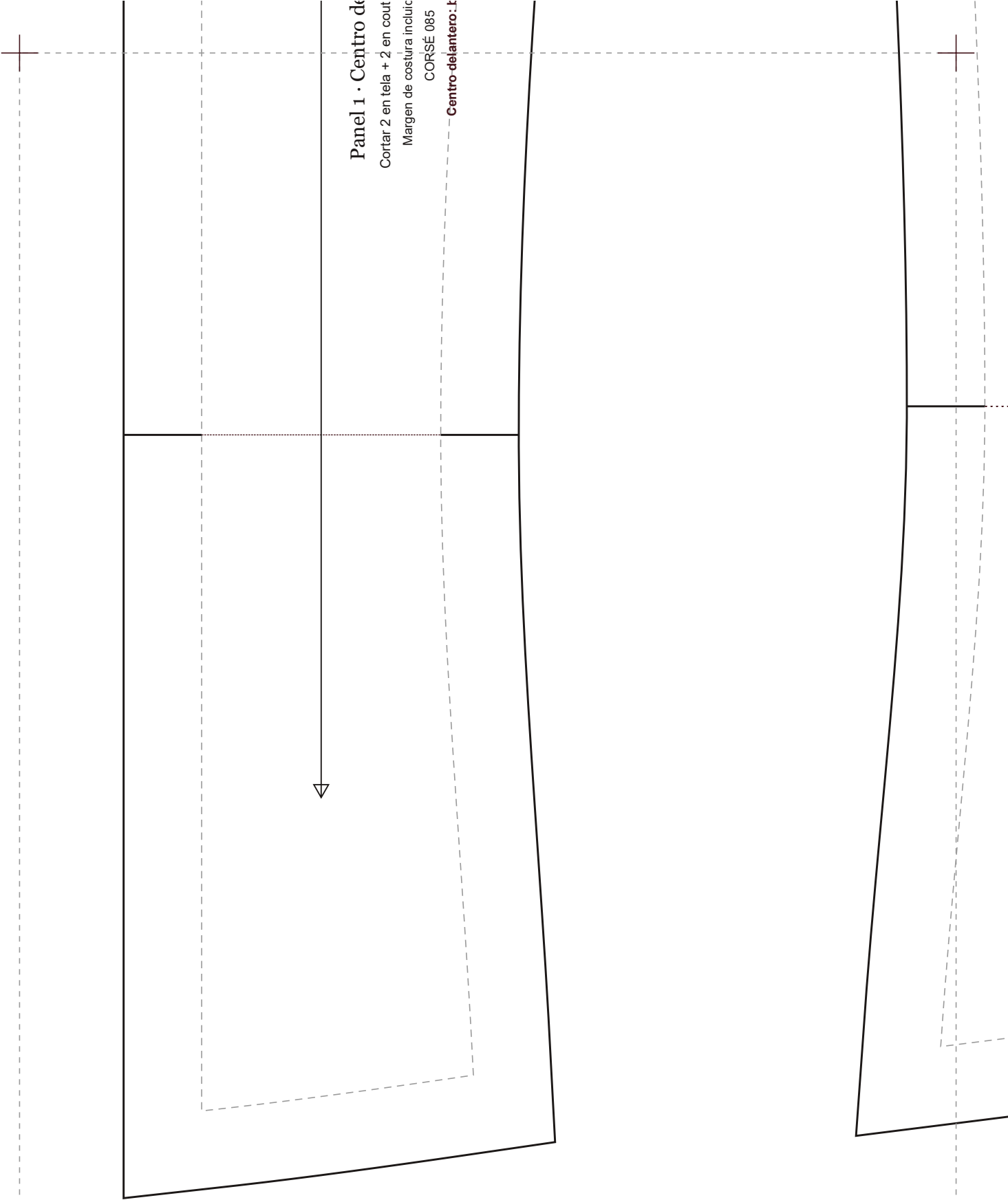
CORSÉ 085 · Sobre Busto Escote en V Suave · 7 Paneles · escala 1:1 · 93,3 × 48,7 cm
