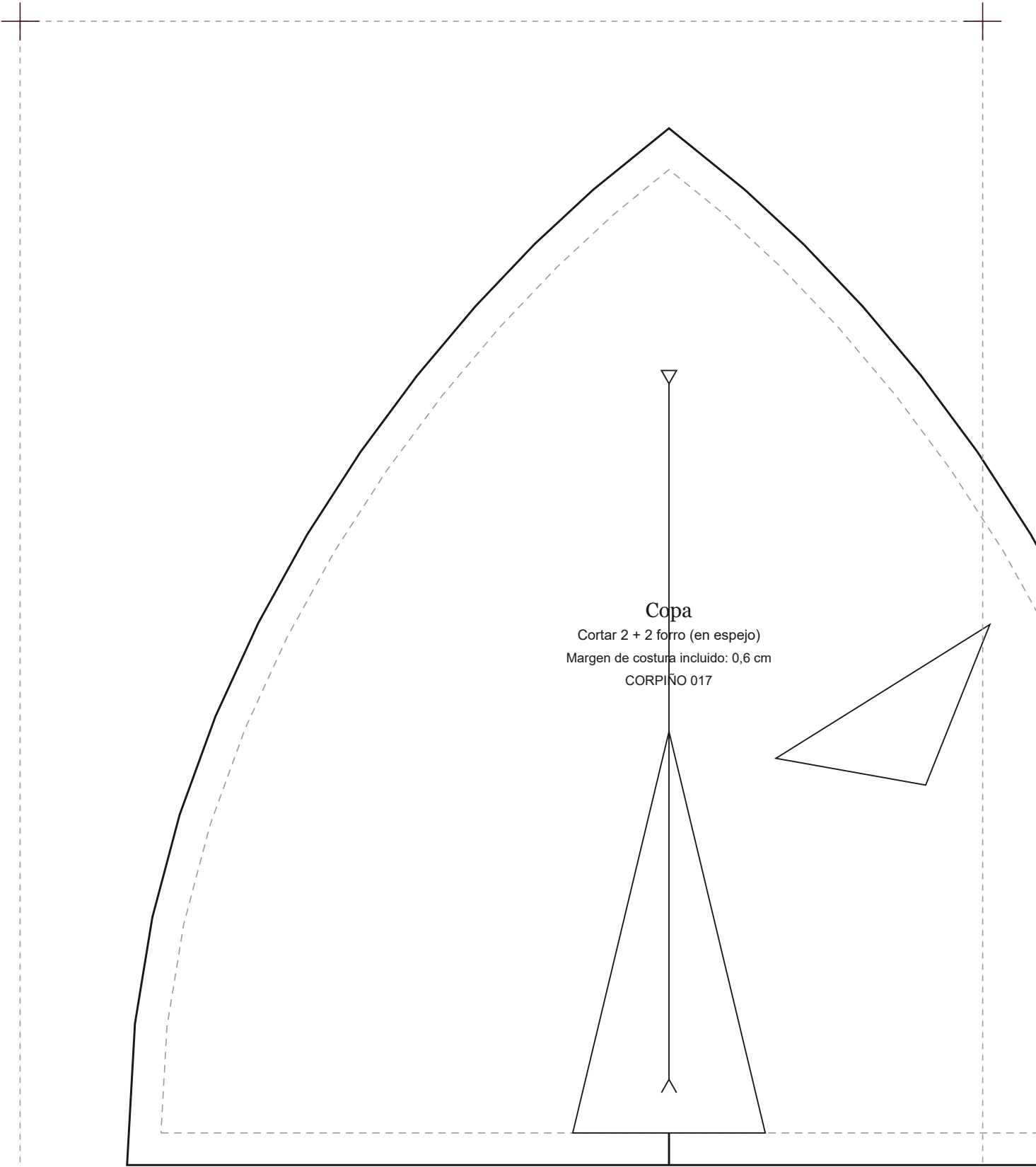
CORPIÑO 017 · Corpiño de Copa Entera sin Aro · escala 1:1 · 60,7 × 23,4 cm
