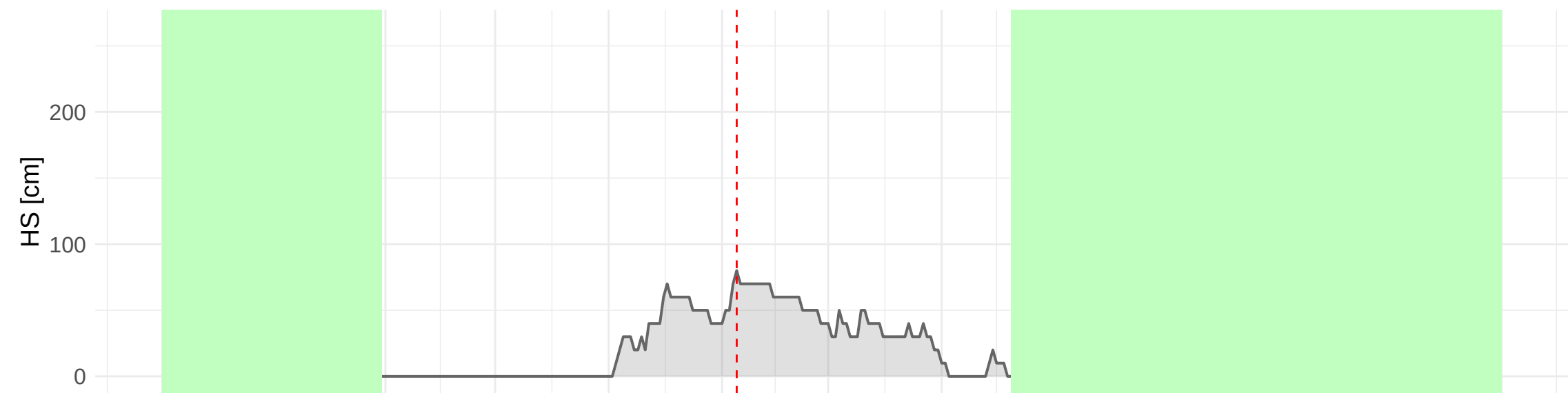
HSD_TAA_TN_MONTE_BONDONE_VIOTE_MAN (1490 m a.s.l.) – 2007 to 2008
