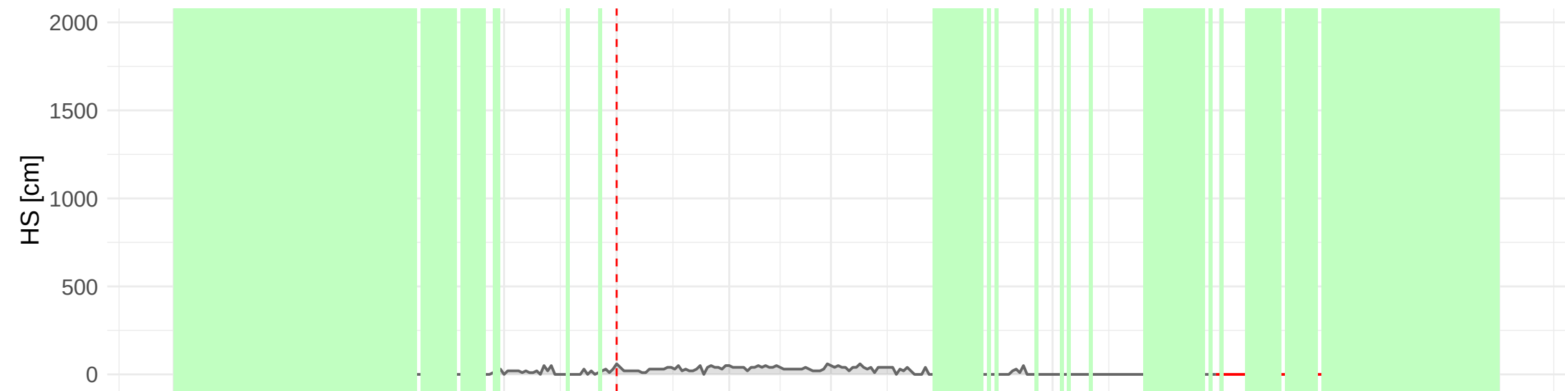
HSD_TAA_TN_PASSO_BROCON_MAN (1610 m a.s.l.) – 2000 to 2001
