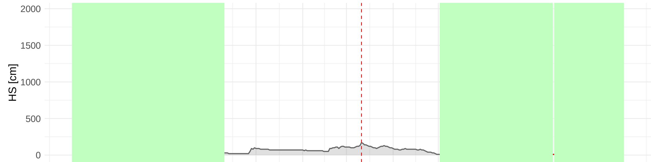
HSD_TAA_TN_PASSO_BROCON_MAN (1610 m a.s.l.) – 2003 to 2004
