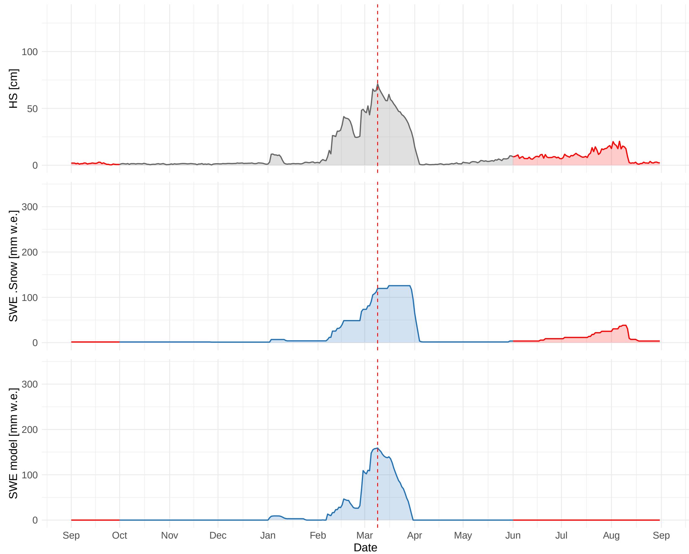
HSD_TAA_TN_PASSO_SOMMO (1360 m a.s.l.) – 2015 to 2016
