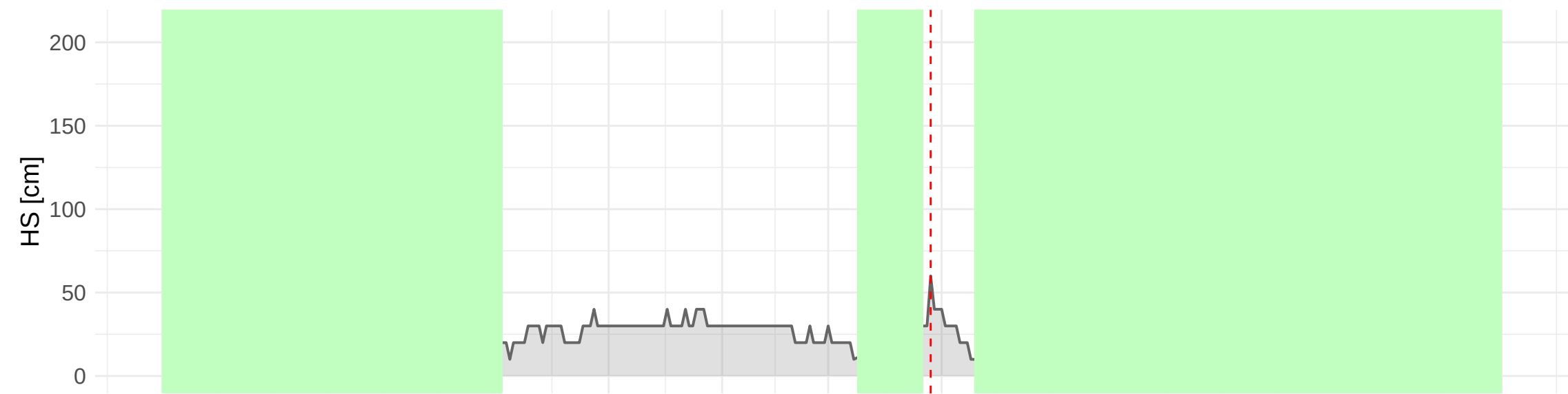
HSD_TAA_TN_PASSO_SOMMO_MAN (1360 m a.s.l.) – 1999 to 2000
