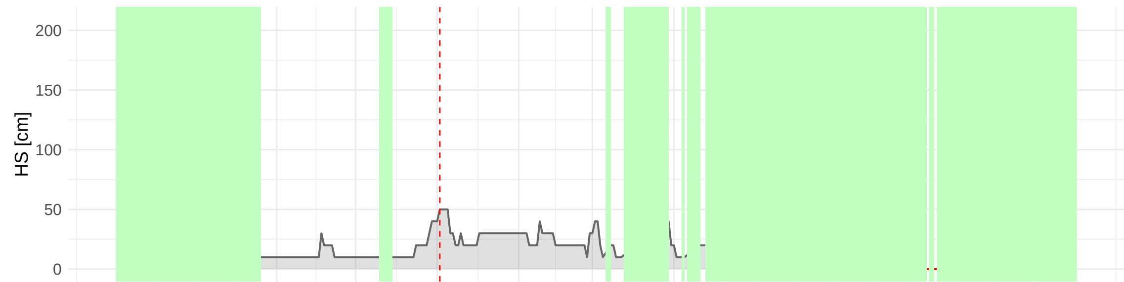
HSD_TAA_TN_PASSO_SOMMO_MAN (1360 m a.s.l.) – 2000 to 2001
