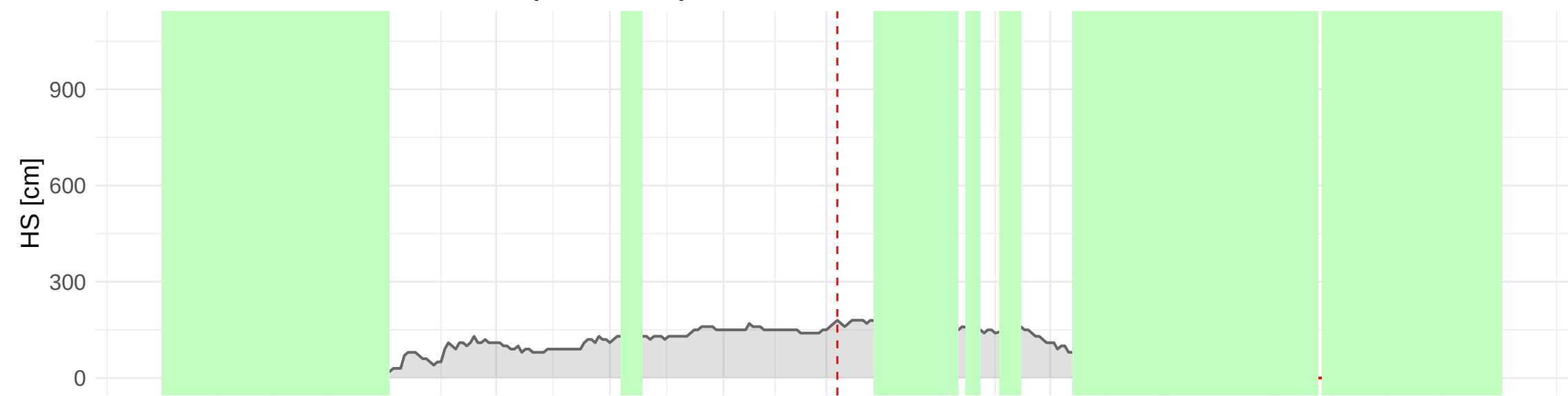
HSD_TAA_TN_PASSO_TONALE_MAN (1875 m a.s.l.) – 2000 to 2001
