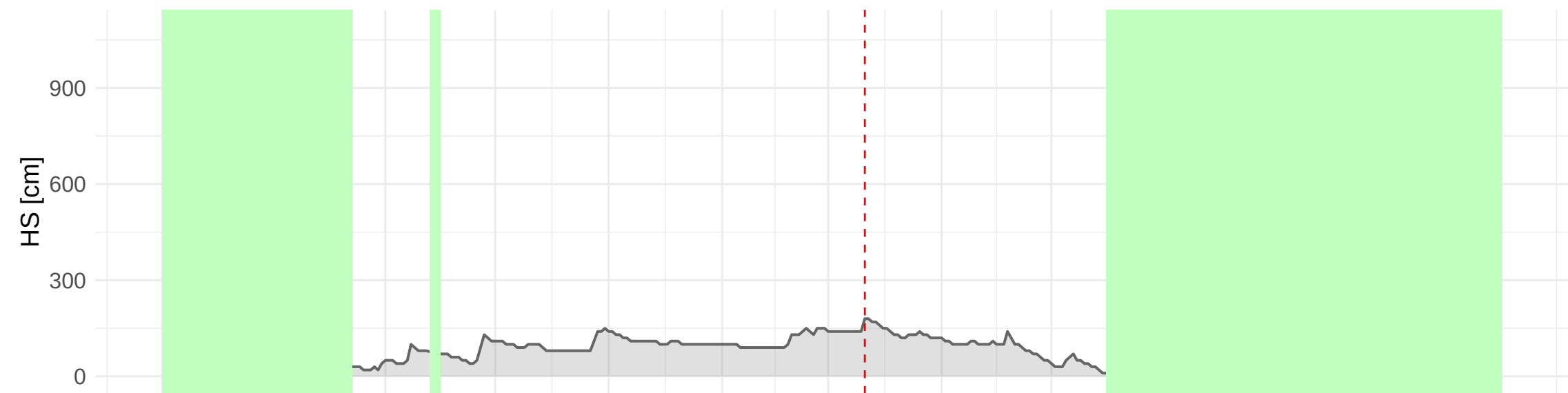
HSD_TAA_TN_PASSO_TONALE_MAN (1875 m a.s.l.) – 2003 to 2004
