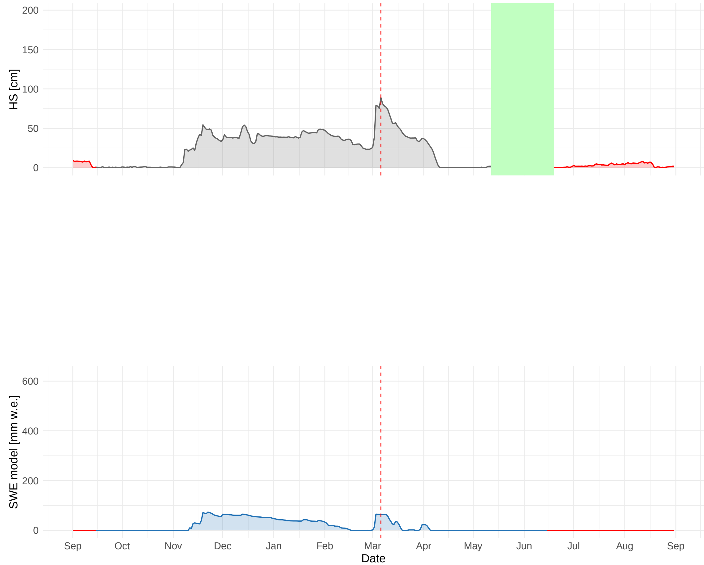
HSD_TAA_TN_TREMALZO (1560 m a.s.l.) – 2019 to 2020
