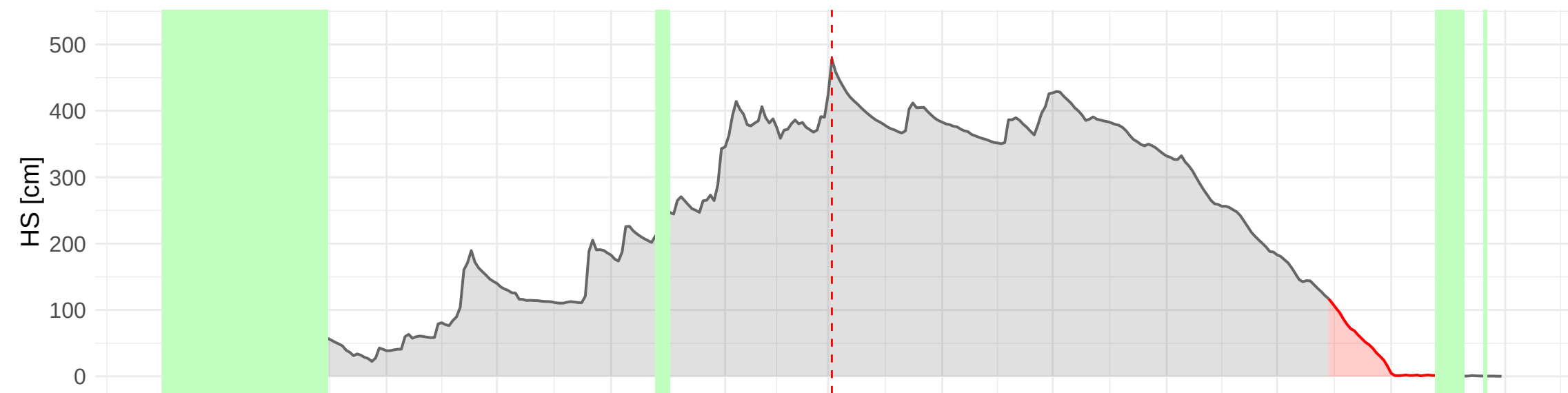
HSD_TAA_TN_VERMIGLIO_CAPANNA_PRESENA (2715 m a.s.l.) – 2013 to 2014
