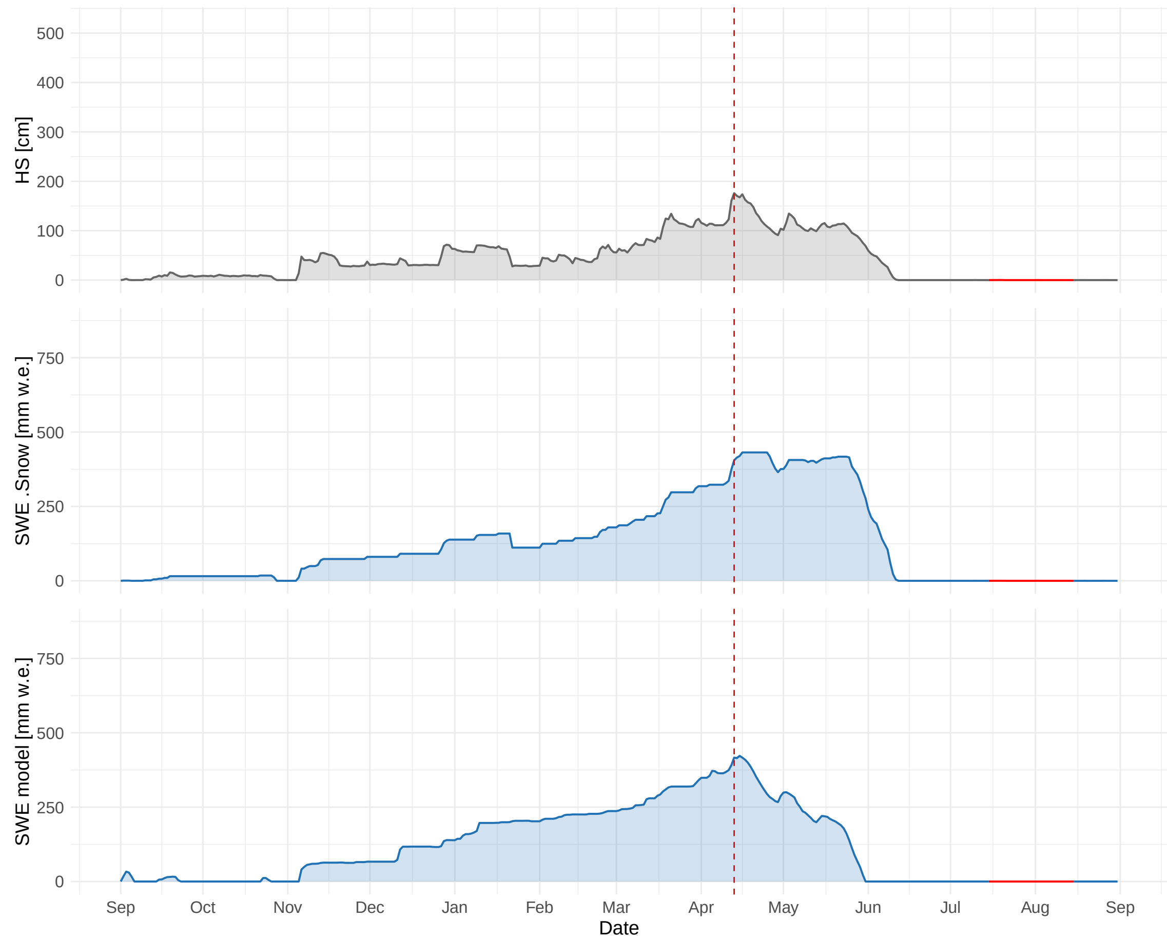
HSD_TAA_TN_VERMIGLIO_CAPANNA_PRESENA (2715 m a.s.l.) – 2017 to 2018
