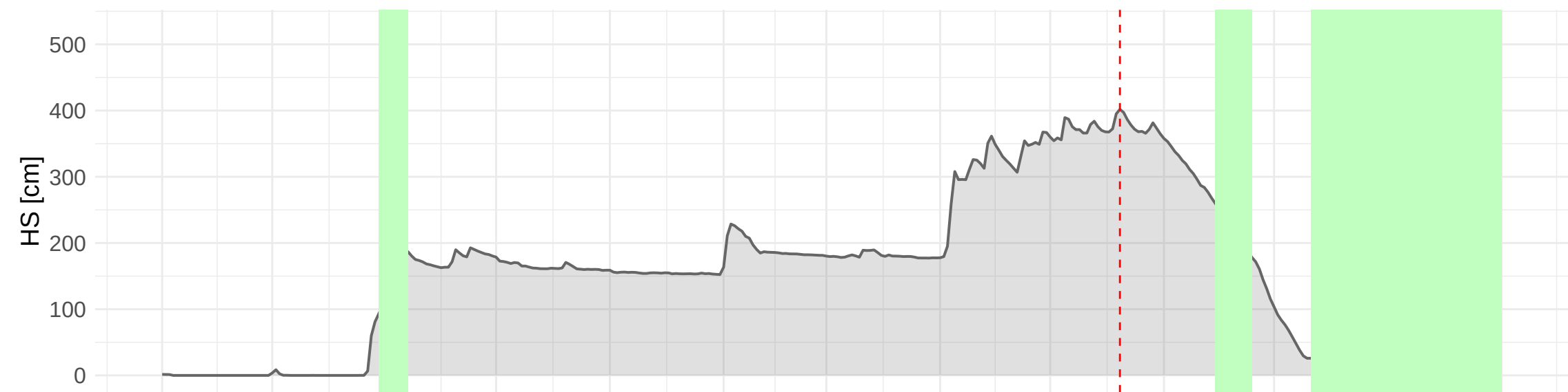
HSD_TAA_TN_VERMIGLIO_CAPANNA_PRESENA (2715 m a.s.l.) – 2018 to 2019
