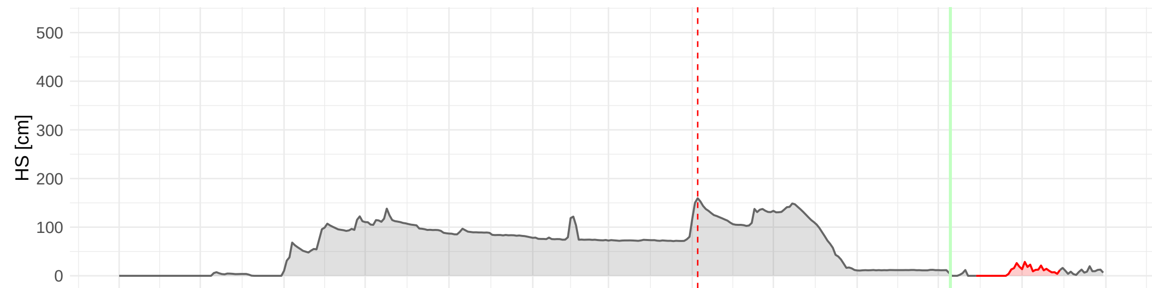
HSD_TAA_TN_VERMIGLIO_CAPANNA_PRESENA (2715 m a.s.l.) – 2021 to 2022
