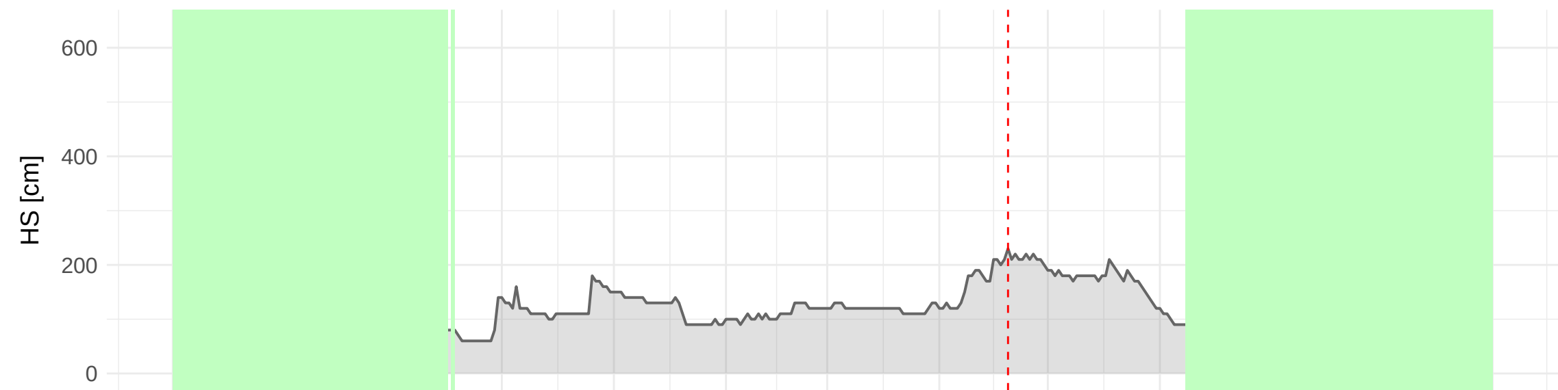
HSD_TAA_TN_VERMIGLIO_CAPANNA_PRESENA_MAN (2715 m a.s.l.) – 2004 to 2005
