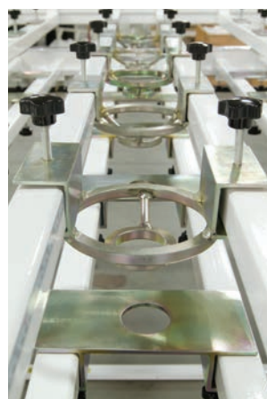
Compression rings Anillos de compresión
