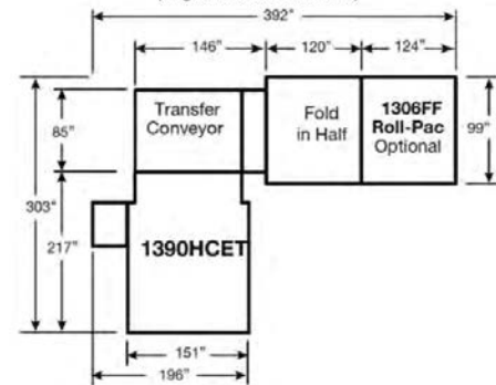
Left or Right Angle Configuration (Right Angle illustrated) Configuración del Angulo Derecho o Izquierdo (Angulo Derecho Ilustrado)
