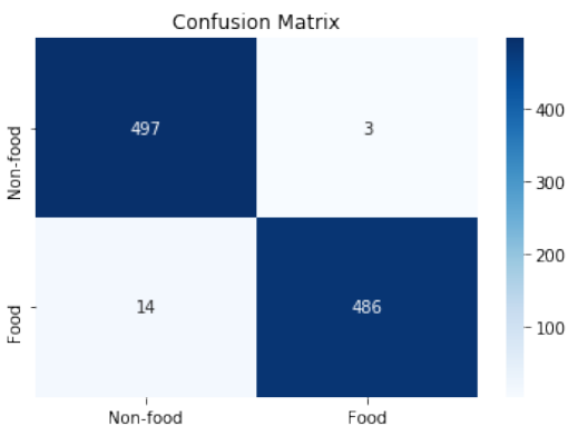
Hình 3.4: Confusion Matrix
