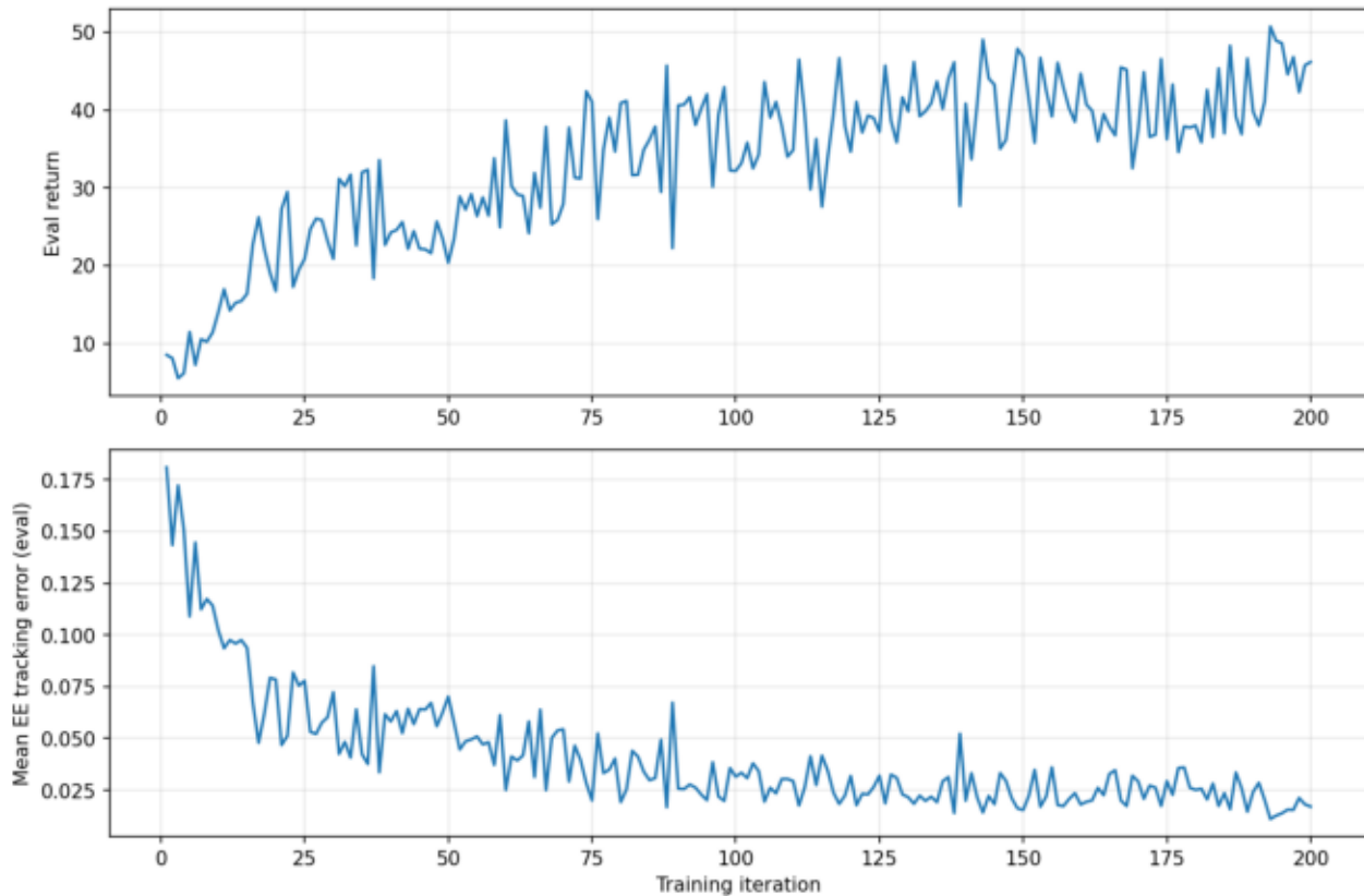
PPO (26_04_16_20_46_14_model)
