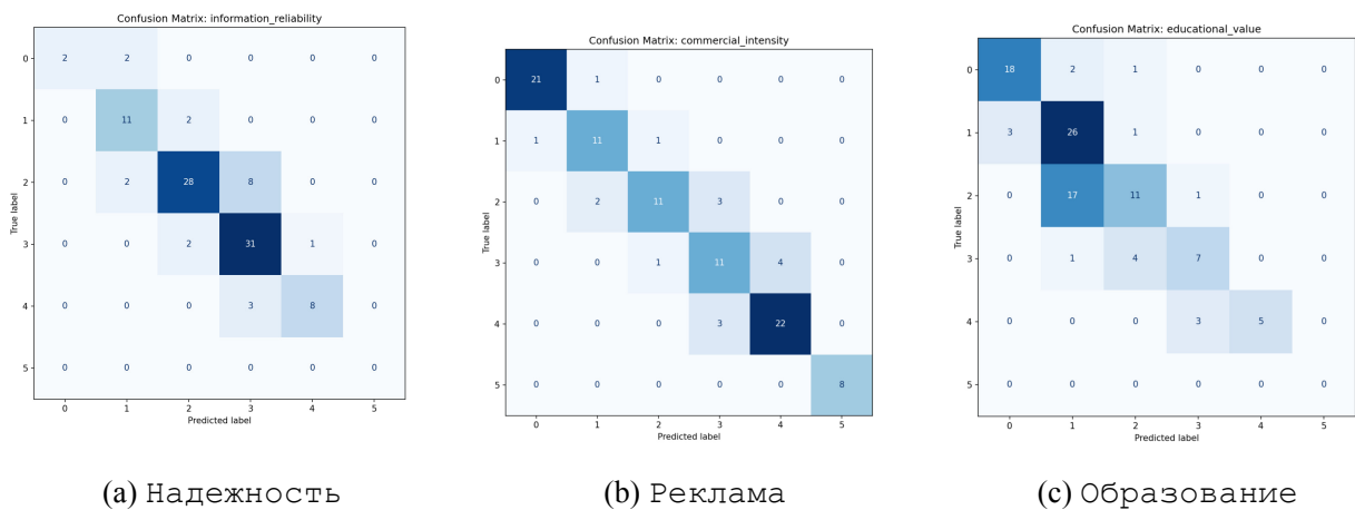
Рис. 3: Матрицы ошибок модели RuModernBERT
