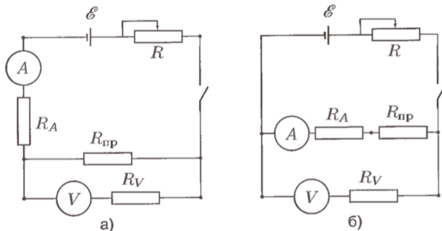
Figure 1: Схемы для измерения сопротивления при помощи амперметра и вольтметра
