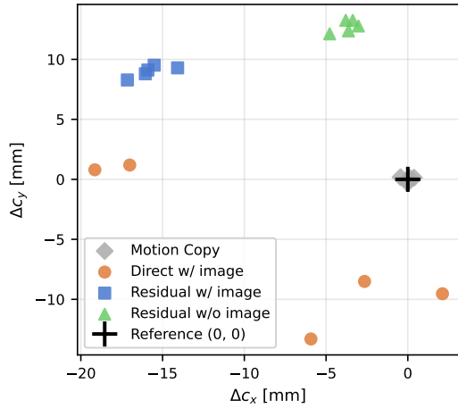
図 3: c = [0, 0] 時のプレース位置分布 (ラベル座標系). + はモーションコピーの平均位置 (基準点 (0, 0)) を示す.
