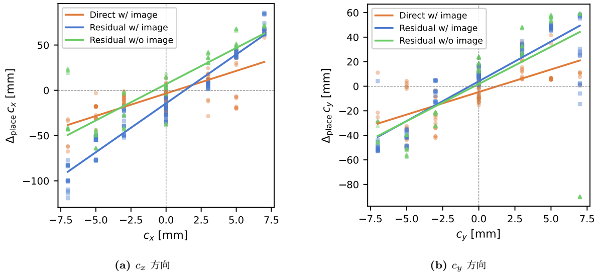
図 1: ラベルとプレース変位の関係（各モデルの散布図と回帰直線）
