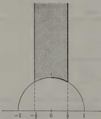
FIG. 7-2. \tau -plane.
