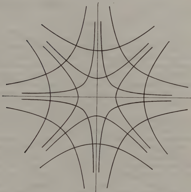
FIG. 3-5. z -plane.
