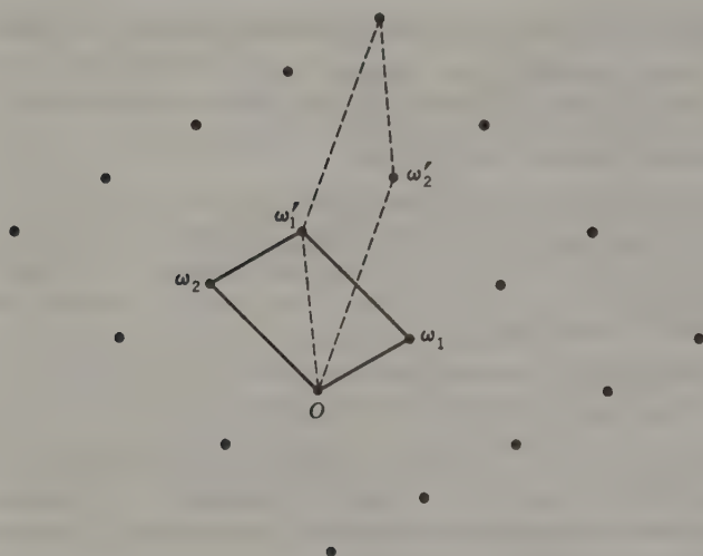
FIG. 7-1. Period module.
