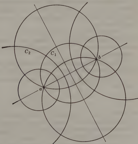
FIG. 3-3. Steiner circles.
