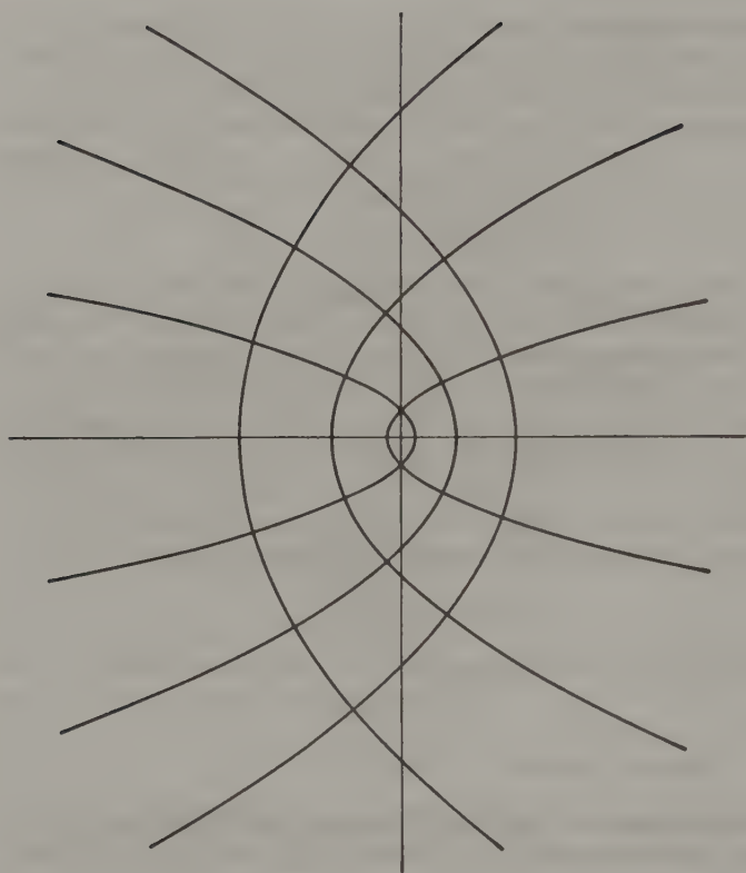
FIG. 1-6. w -plane.
