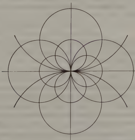
FIG. 3-4. Degenerate Steiner circles.
