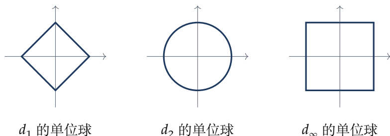
图 2.1: \mathbb{R}^2 上三个度量的单位球 \{x \mid d(x, 0) \leq 1\} 。同一个集合配上不同的度量,「离原点不超过 1 的点」构成的形状完全不同。这三个度量将在习题 2.4 中被证明是等价的,即它们给出相同的开集与相同的收敛数列。
