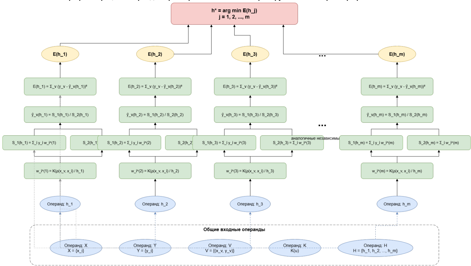
Граф «операции–операнды»: распараллеливание по перебору значений параметра размытости h
