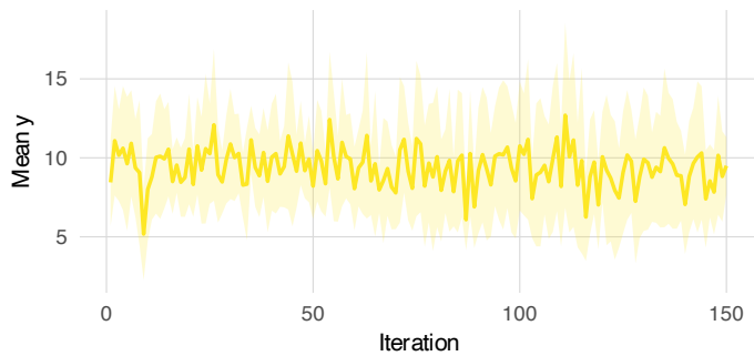
BOCS-SDP
