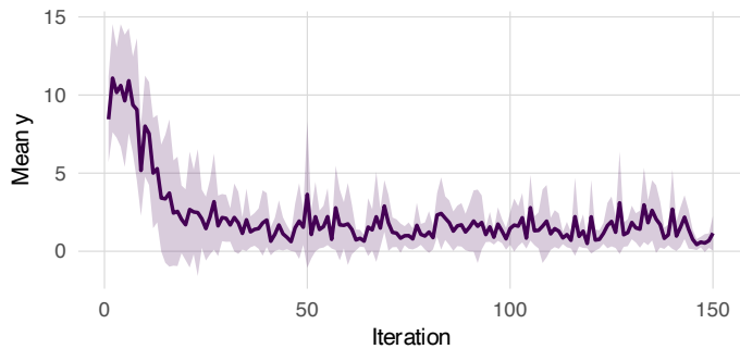
VaRCBO-GA
