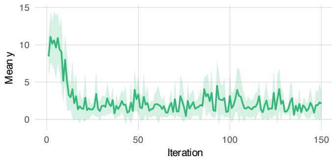
BOCS-GA
