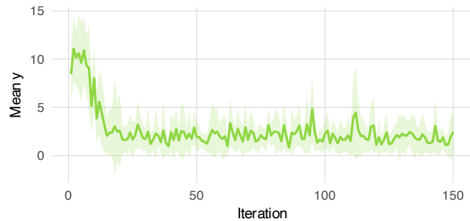
BOCS-SA
