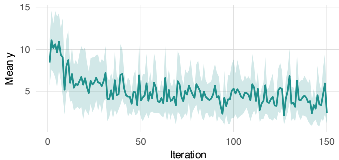
BOCS-SDP
