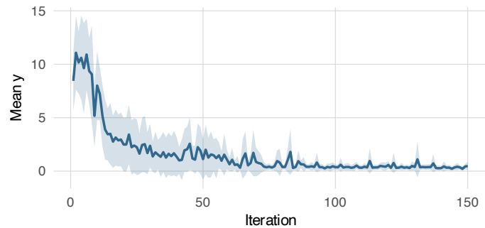
BOCS-SA
