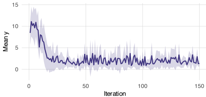
BOCS-GA
