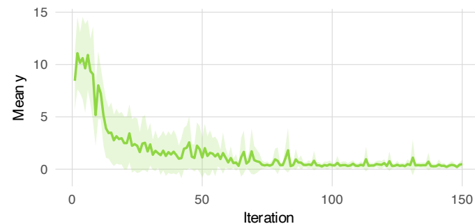
VaR-CBO-BFGS
