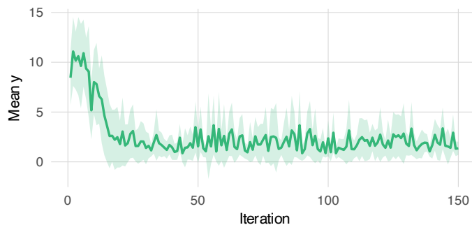
PRCBO-GA
