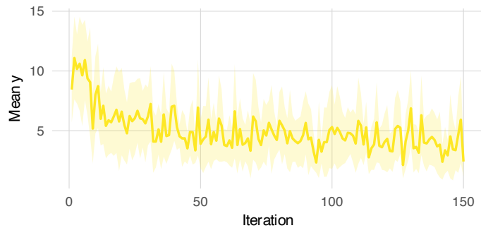
VaR-CBO-GA
