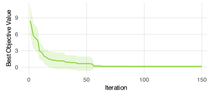
VaR-CBO-BFGS
