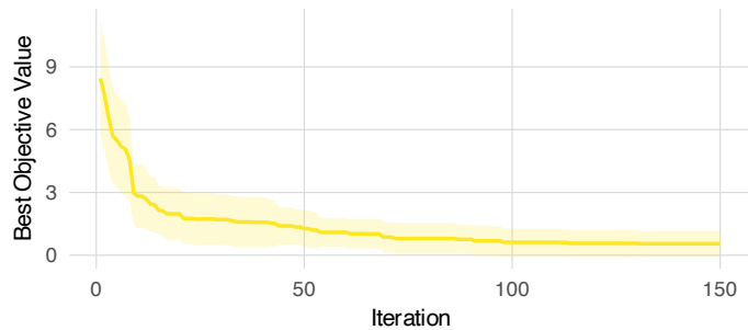
VaR-CBO-GA
