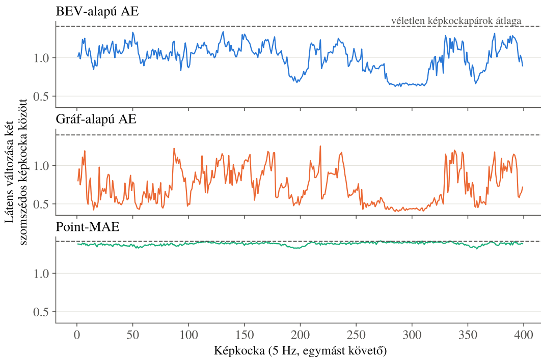
13. ábra. A látens változása 400 egymást követő képkockán; a szaggatott vonal két véletlen képkocka látensének átlagos távolsága
