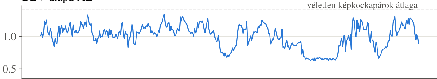
Gráf-alapú AE
