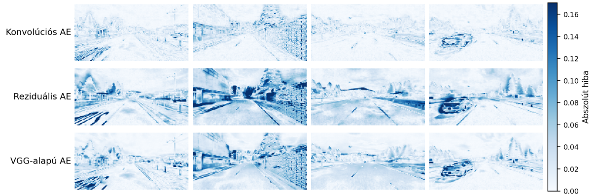
7. ábra. A rekonstrukciók abszolút hibája képpontonként, közös skálán (sötétebb = nagyobb hiba)
