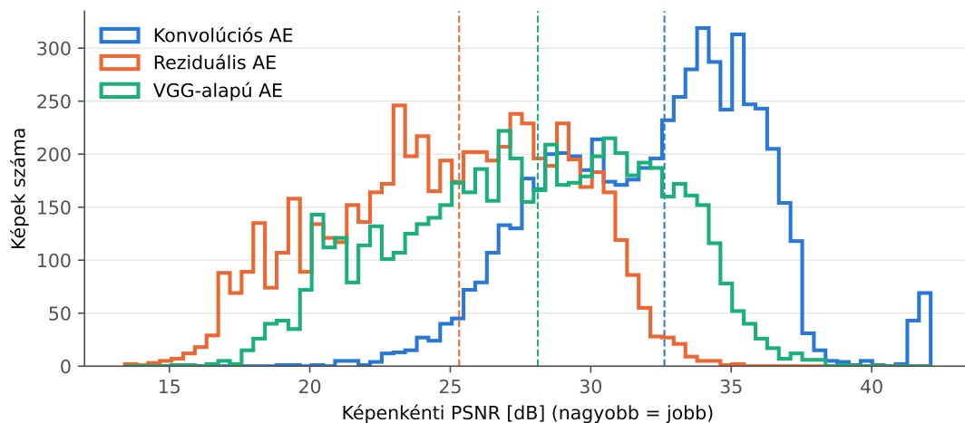
8. ábra. A képenkénti PSNR eloszlása a teszhalmazon; a szaggatott vonalak a modellek mediánját jelölik
