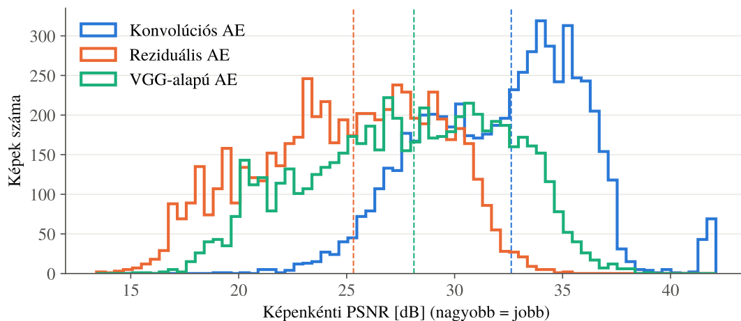
8. ábra. A képenkénti PSNR eloszlása a tesztalmazon; a szaggatott vonalak a modellek mediánját jelölik
