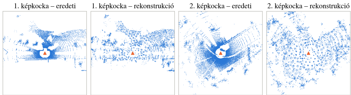
12. ábra. A Point-MAE rekonstrukciói felülnézetből (a háromszög a saját jármű)
