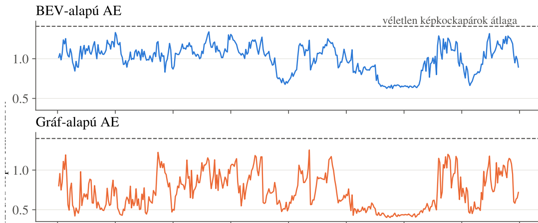
13. ábra. A látens változása két szomszédos képkocka között, 400 egymást követő képkockán (5 Hz); a szaggatott vonal két véletlen képkocka látensének átlagos távolsága
