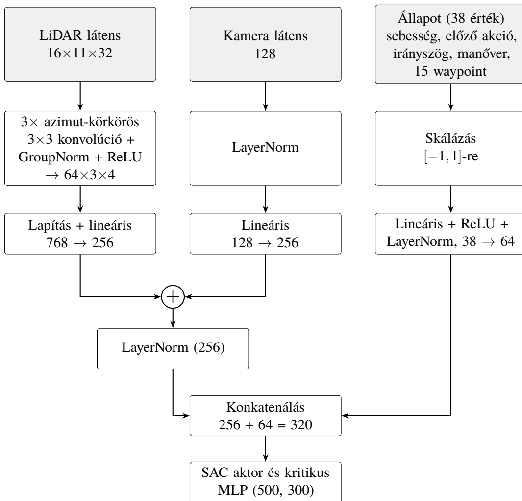
14. ábra. A saját jellemzőkinyerő felépítése; a szürke dobozok a bemenetek
