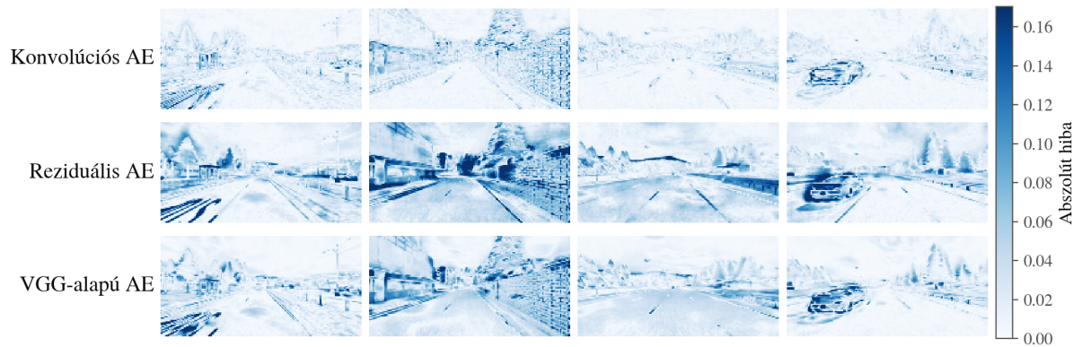
7. ábra. A rekonstrukciók abszolút hibája képpontonként, közös skálán (sötétebb = nagyobb hiba)
