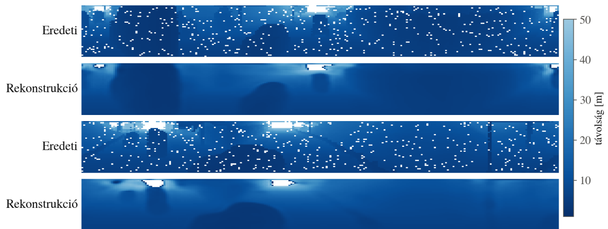
11. ábra. A gráf-alapú autoenkóder rekonstrukciói két képkockán (sötétebb = közelebb, fehér = nincs visszaverődés)
