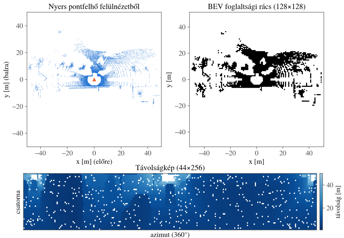
9. ábra. Ugyanaz a LiDAR-képkocka a három modell bemeneti formájában; a háromszög a saját járművet jelöli, a távolságképen a fehér cellákból nem érkezett visszaverődés
