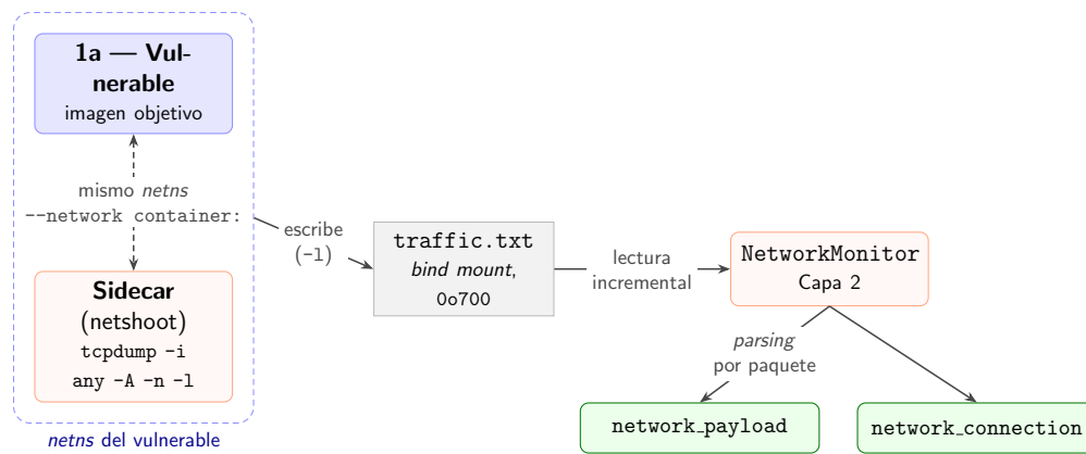
Figura 4.1: Pipeline de captura de red: tcpdump escribe traffic.txt en un bind mount desde el netns del vulnerable. El monitor emite network_payload y network_connection .
