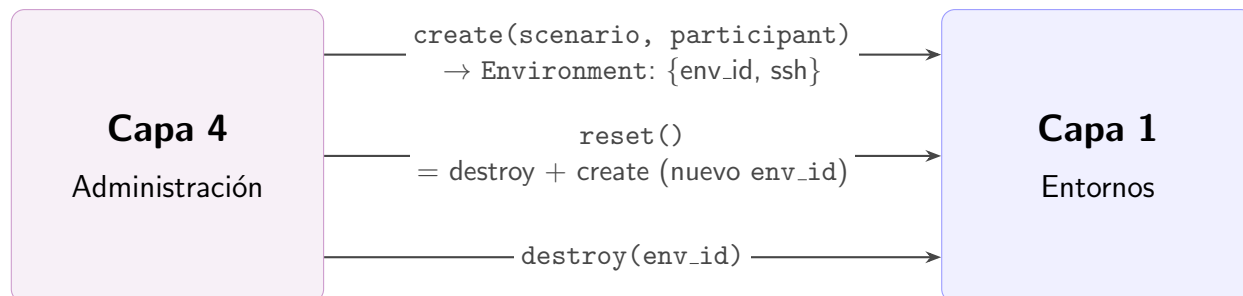
Figura 3.5: Contrato Capa 4 → Capa 1: ciclo de vida vía EnvironmentProvider .
