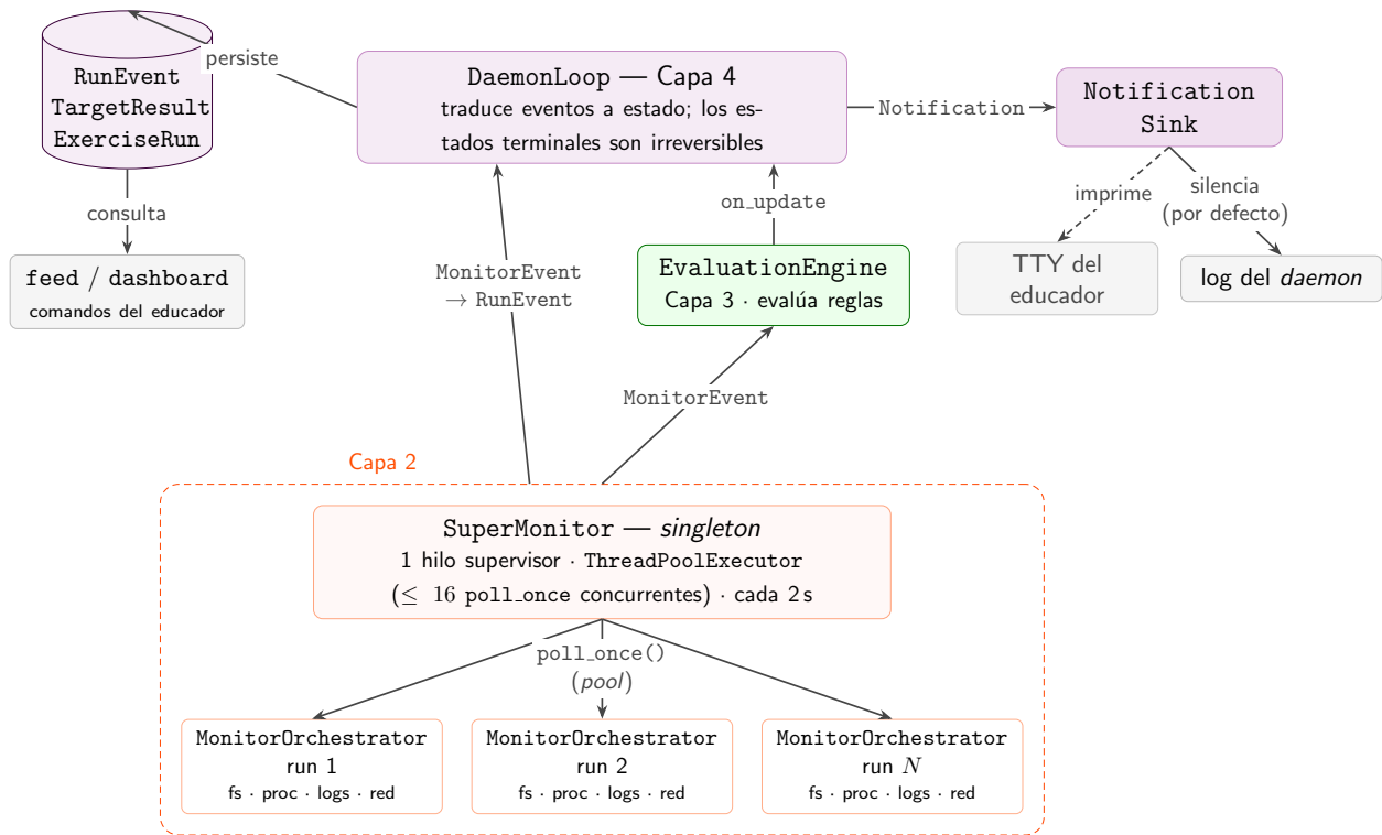
Figura 4.2: Componentes del daemon: DaemonLoop y SuperMonitor (con su ThreadPoolExecutor) coordinan N MonitorOrchestrator y los cuatro monitores; el flujo de MonitorEvent pasa por el EvaluationEngine hacia el NotificationSink y la base de datos.
