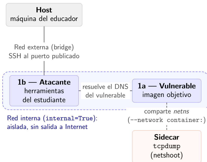
Figura 3.9: Topología de red del entorno: red interna aislada ( internal=True ) y red externa ( bridge ), con el atacante en ambas redes, el vulnerable solo en la interna, y el sidecar compartiendo el netns del vulnerable.
