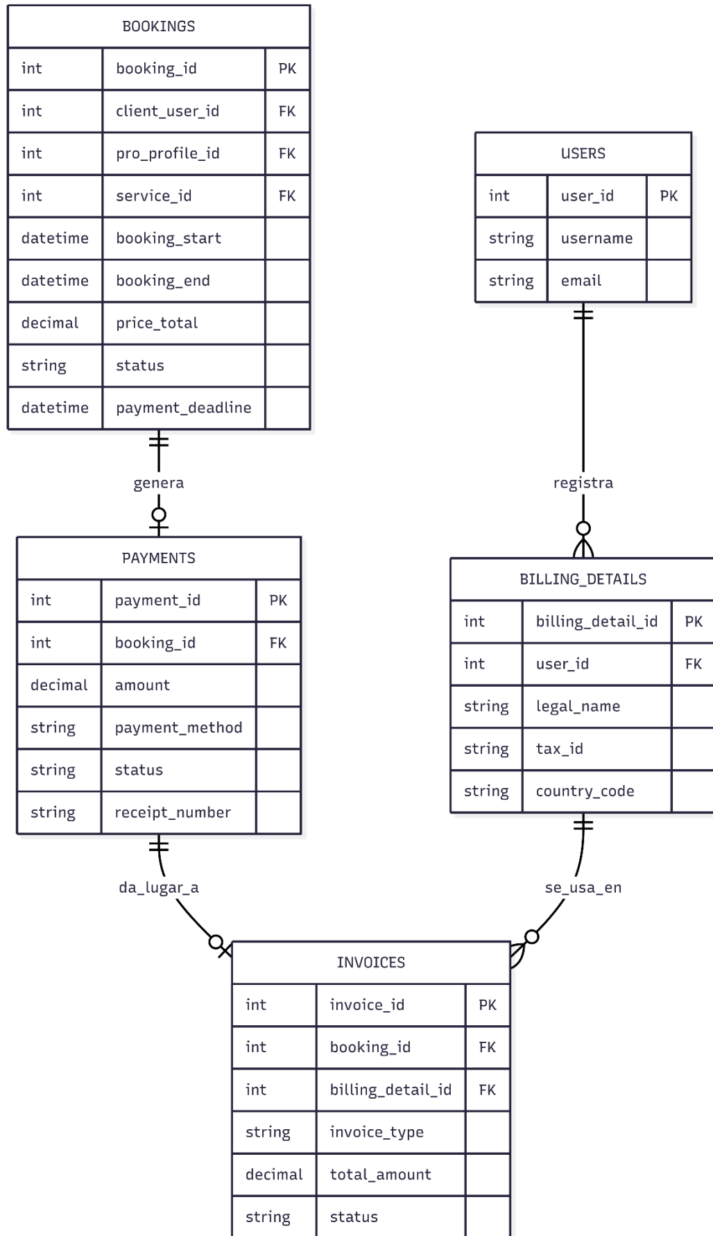
Fig. 4B. Diagrama Entidad-Relación simplificado del sistema del bloque económico. Versión ampliada en este anexo .
