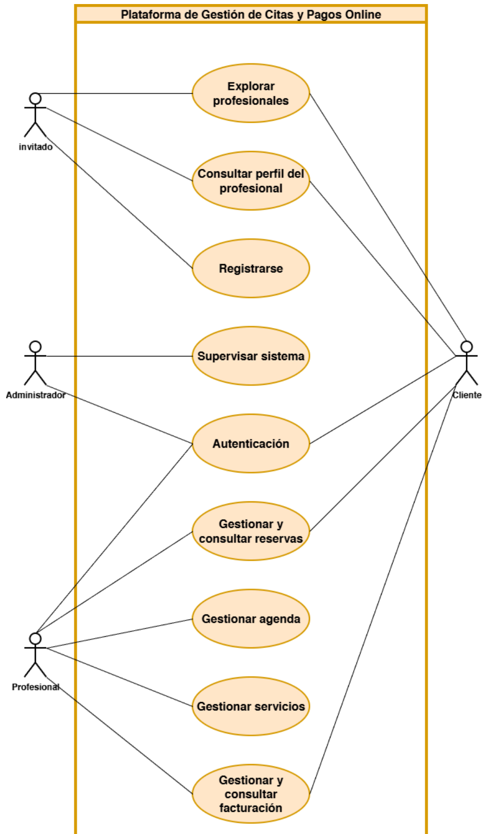
Fig. 1. Diagrama general de los casos de uso principales del sistema.
