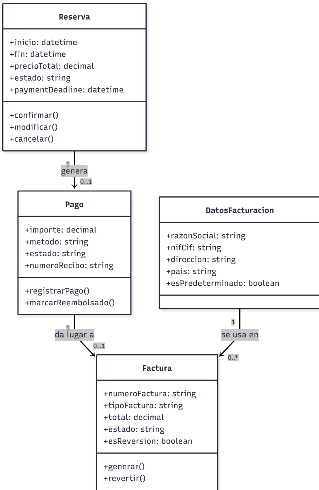
Fig. 2B. Diagrama de clases simplificado del sistema - bloque económico.
