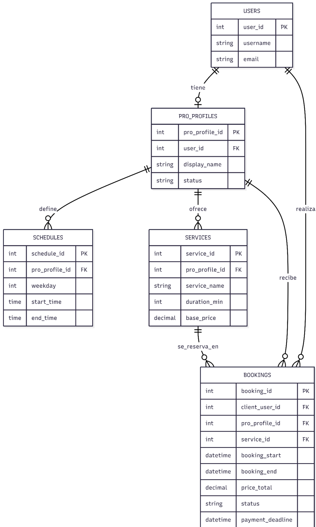
Fig. 4A. Diagrama Entidad-Relación simplificado del sistema del bloque de reservas. Versión ampliada en este anexo .
