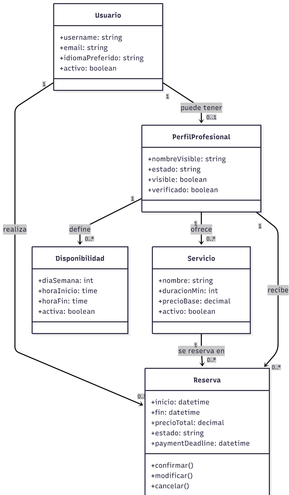
Fig. 2A. Diagrama de clases simplificado del sistema - bloque funcional.
