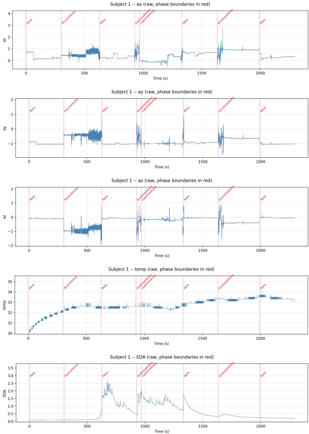
Слика 2: Сирови сигнали записа AccTempEDA (акцелерометар по осама, температура коже, електродермална активност) за Испитаника 1, током целог протокола; вертикалне линије означавају границе фаза.
