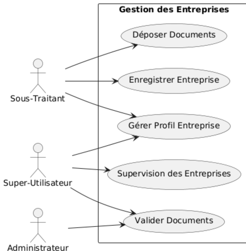
FIGURE 2.3 – Diagramme de Cas d'Utilisation - Gestion des entreprises
