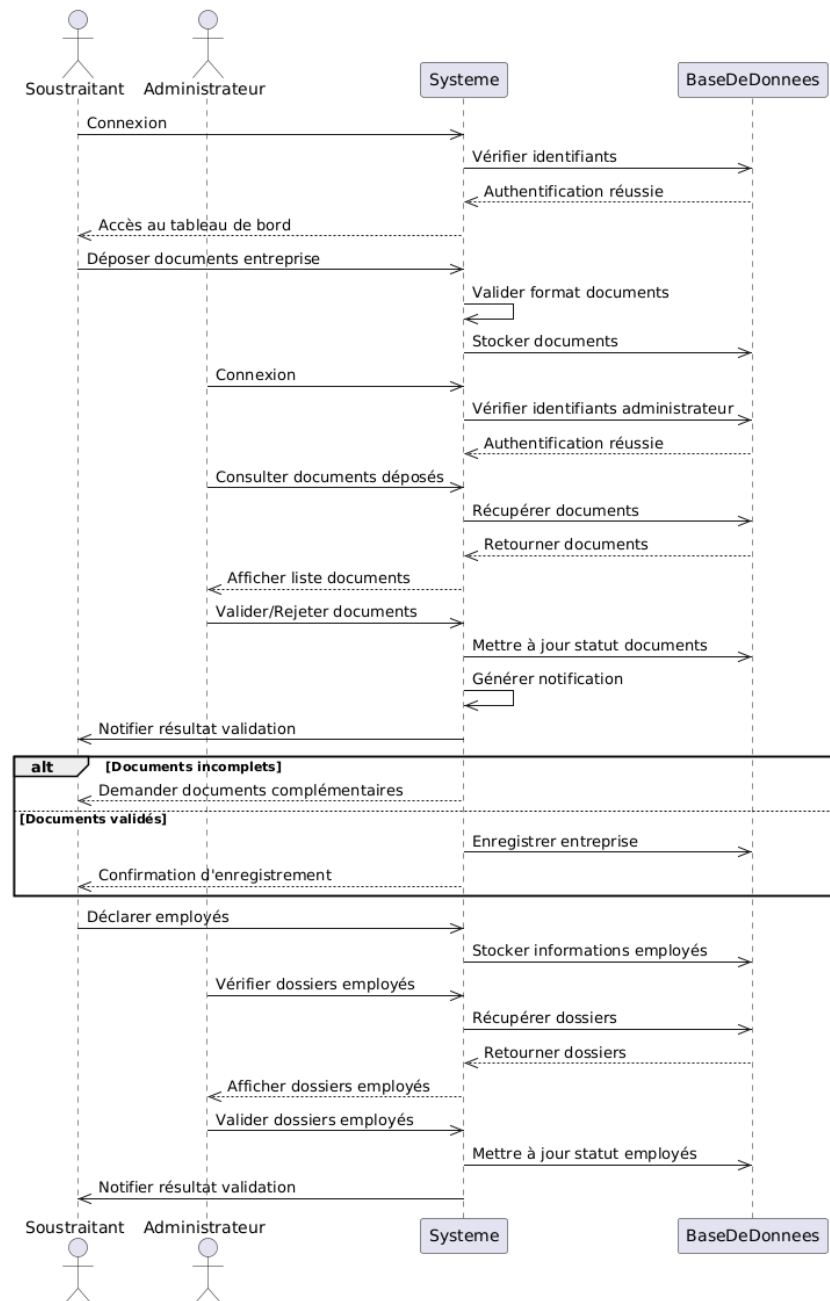
FIGURE 3.7 – Diagramme de séquence global
