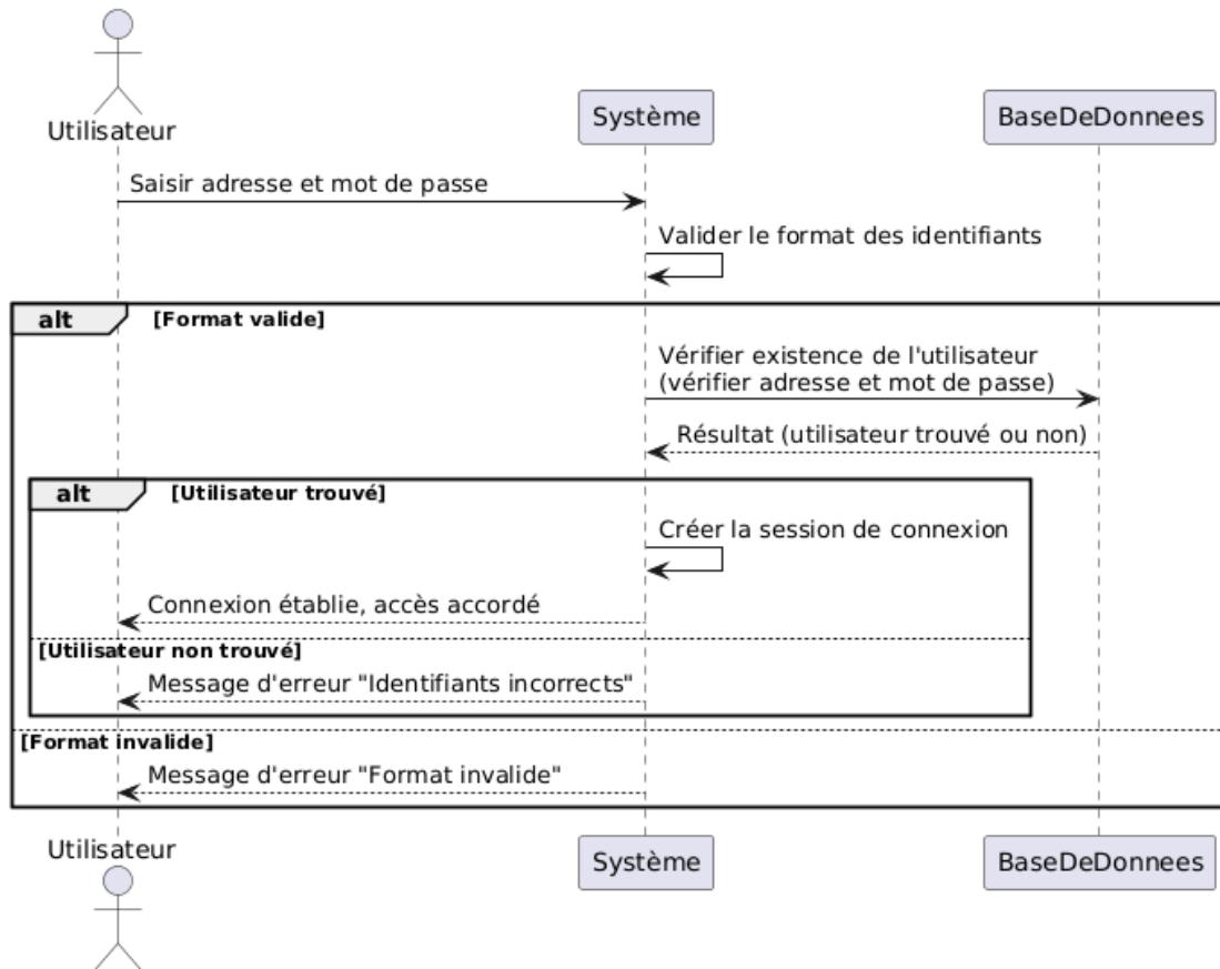
FIGURE 3.8 – Diagramme de Séquence pour l'Authentification
