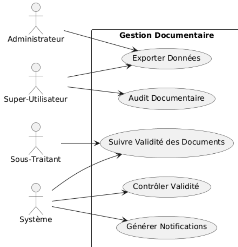
FIGURE 2.5 – Diagramme de Cas d’Utilisation - Gestion Documentaire et Notifications
