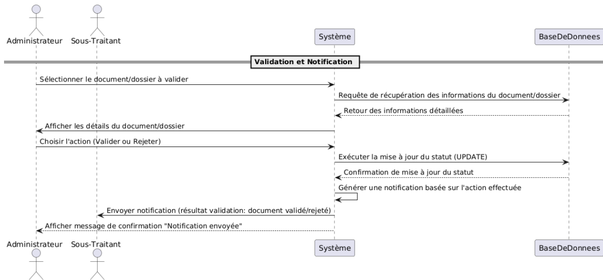
FIGURE 3.11 – Diagramme de Séquence pour la Gestion des Notifications
