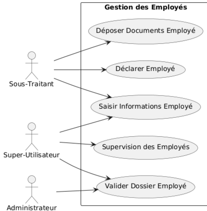
FIGURE 2.4 – Diagramme de Cas d'Utilisation - Gestion des Employés
