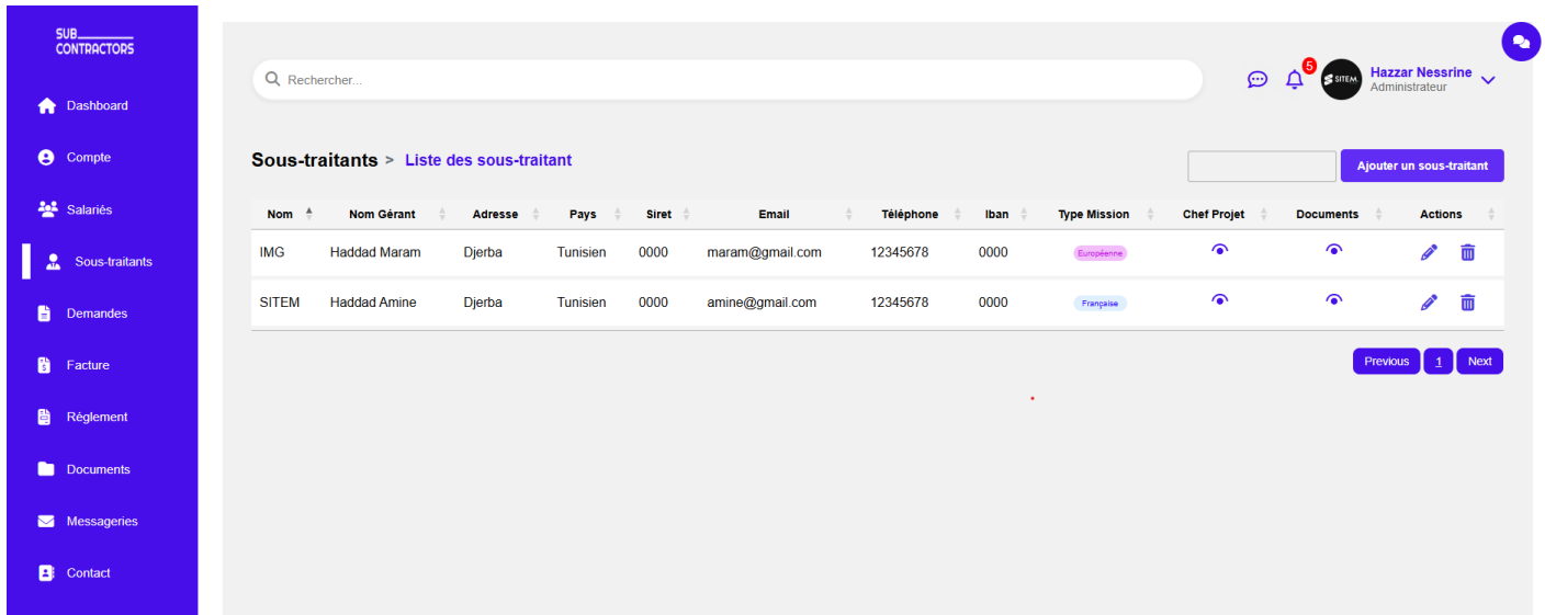
FIGURE 4.8 – Interface Sous-traitants
