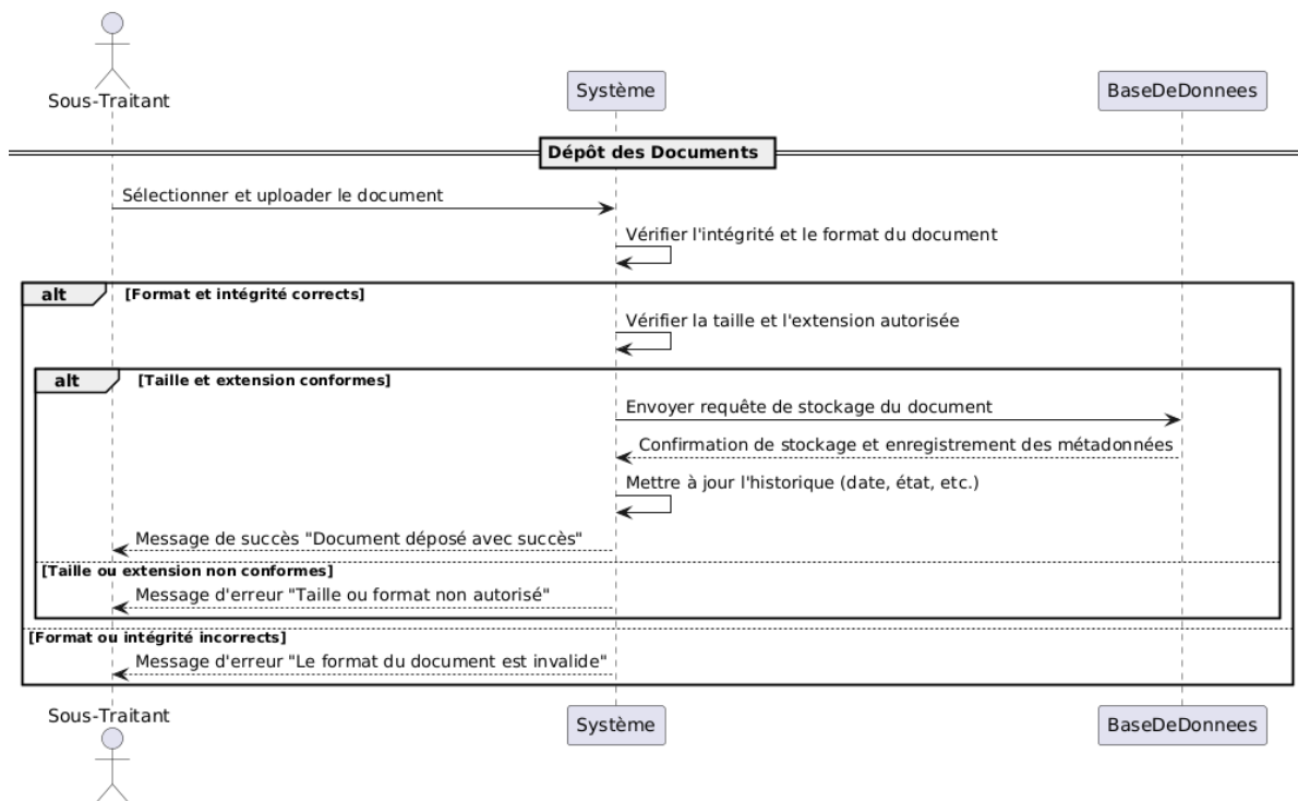
FIGURE 3.10 – Diagramme de Séquence pour le Dépôt des Documents
