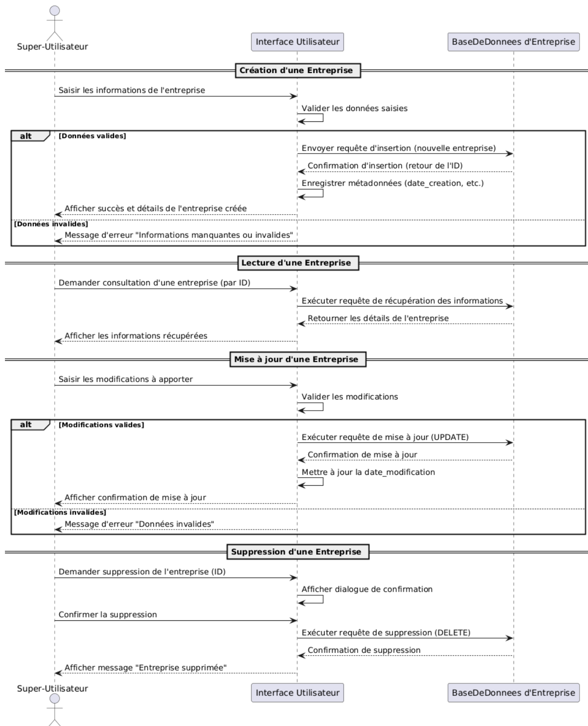
FIGURE 3.9 – Diagramme de Séquence pour les Opérations CRUD du Module Entreprise
