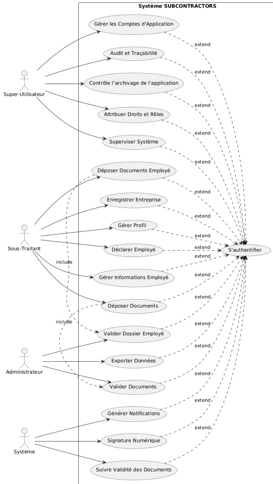
FIGURE 2.1 – Diagramme de Cas d'Utilisation Global
