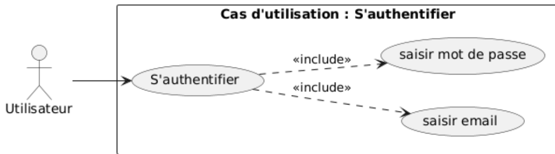
FIGURE 2.2 – Cas d'utilisation : S'authentifier
