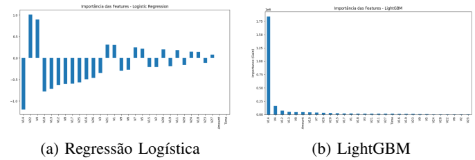
Figura 5: Comparação da importância das variáveis entre Regressão Logística e LightGBM.
