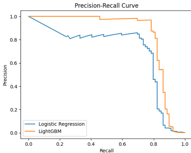
Figura 3: Curva Precision-Recall para Regressão Logística e LightGBM.
