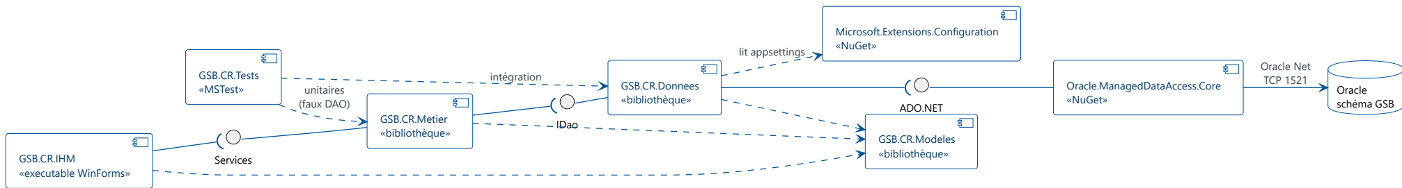
GSB-CR — Diagramme de composants (assemblages .NET et interfaces)
