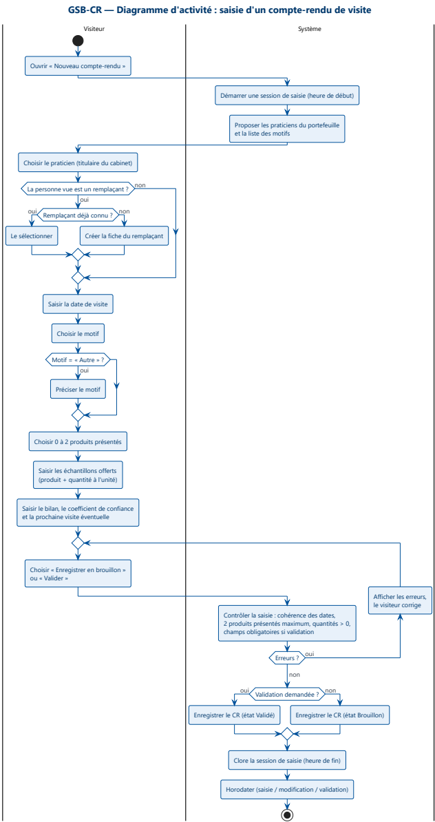
Diagramme 6 — Activité : saisie d'un CR (Comportement · Étapes de la saisie d'un compte-rendu (visiteur / système))
