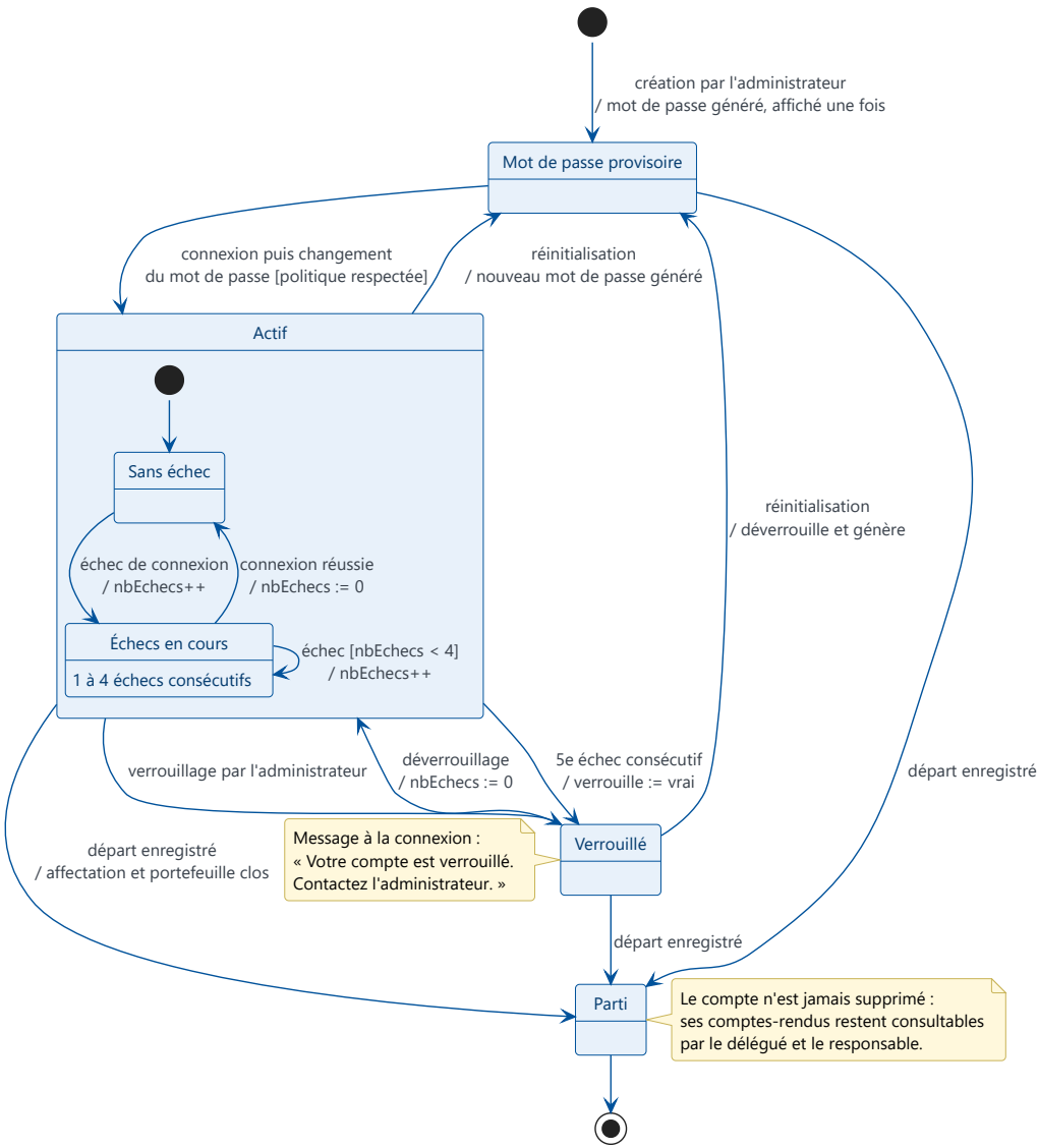
GSB-CR — Diagramme d'états-transitions : compte d'un collaborateur
