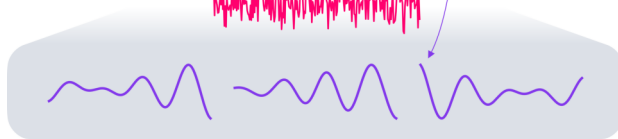
OU process
