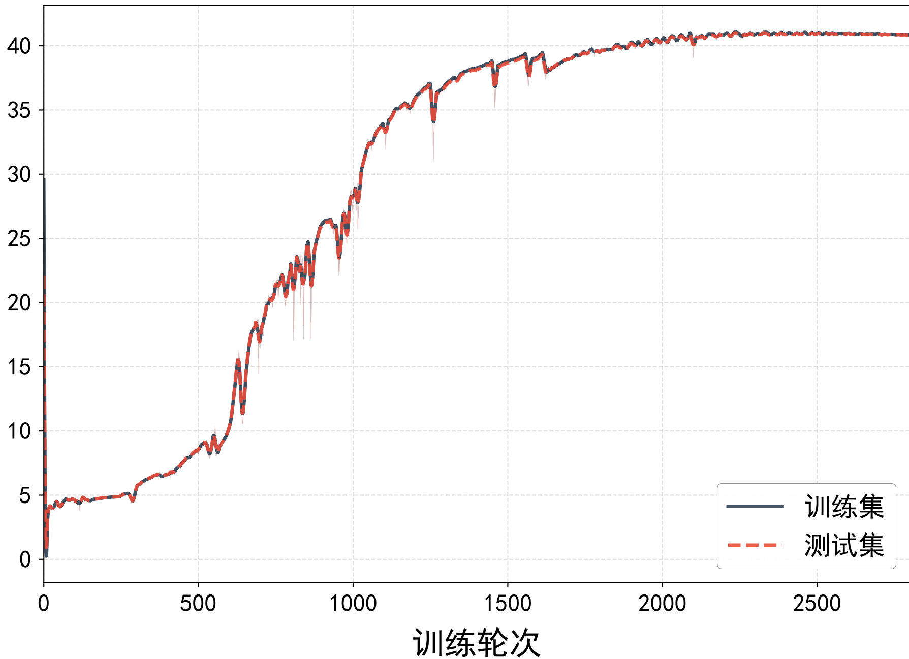
类原型距离
