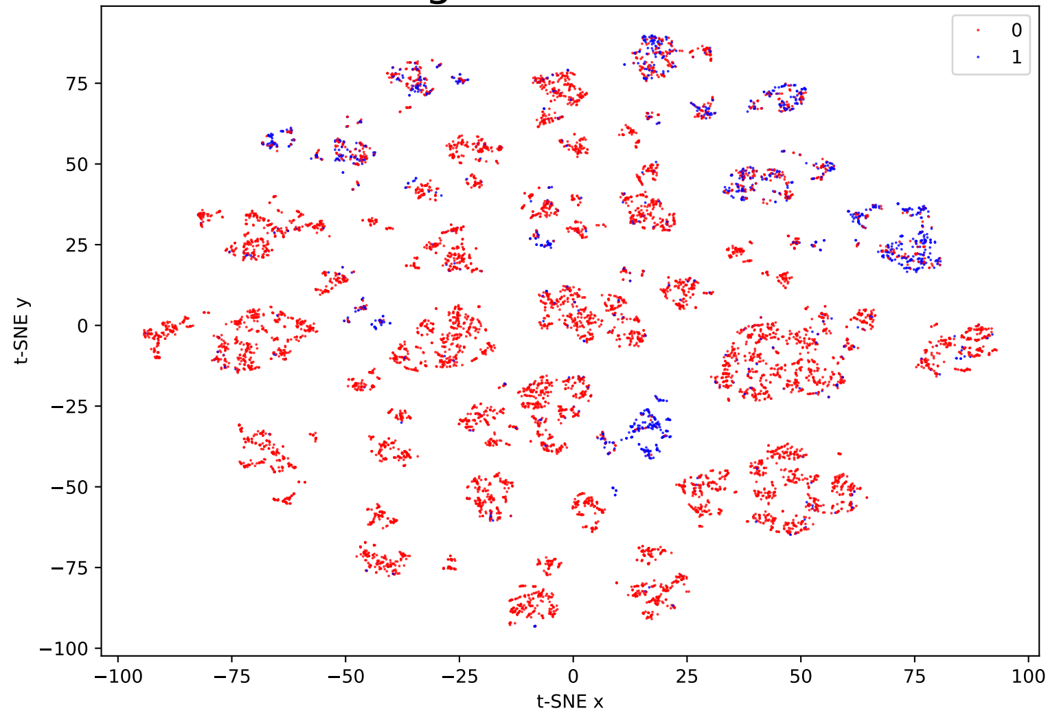
Original data t-SNE
