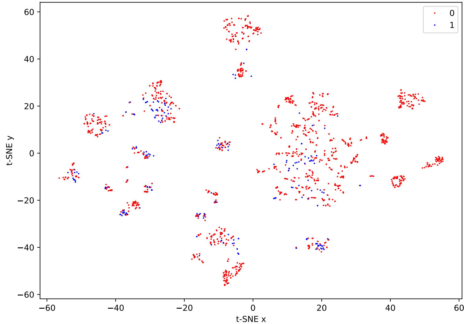
Original data t-SNE
