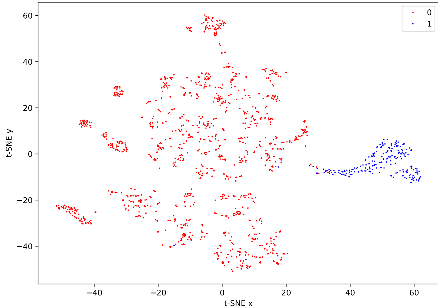
VAE latent data t-SNE
