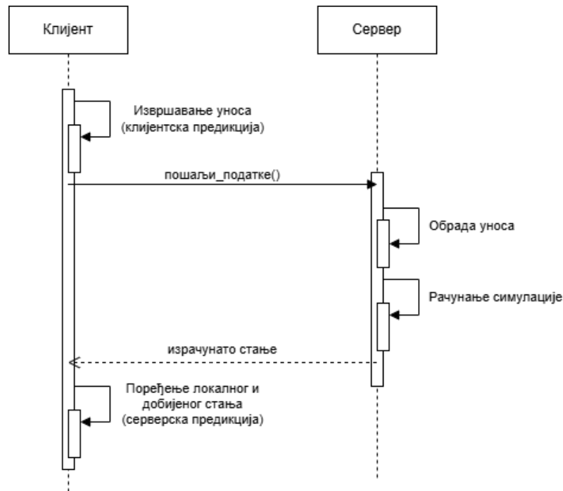
Слика 19: Дијаграм секвенци који приказује ток синхронизације стања.
