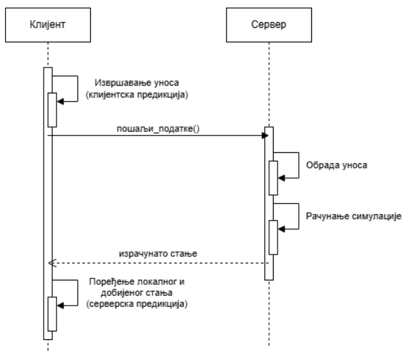
Слика 15: Дијаграм секвенци који приказује ток синхронизације стања.
