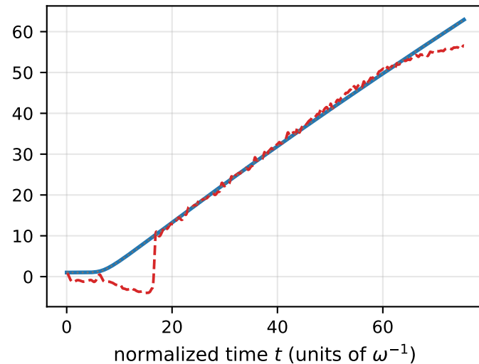
UR ( a_0 = 85 )
